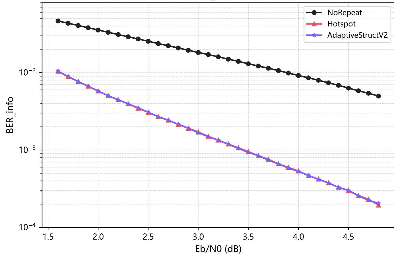
阈值扫描：BER_info随Eb/N0变化
