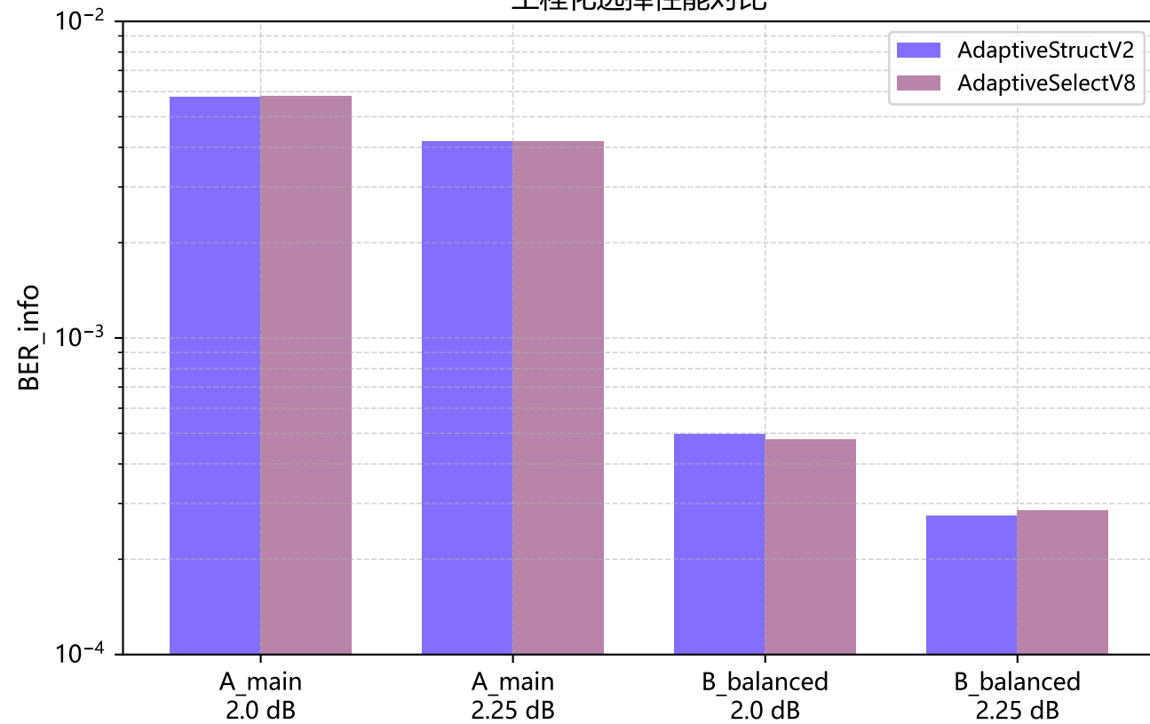
工程化选择性能对比
