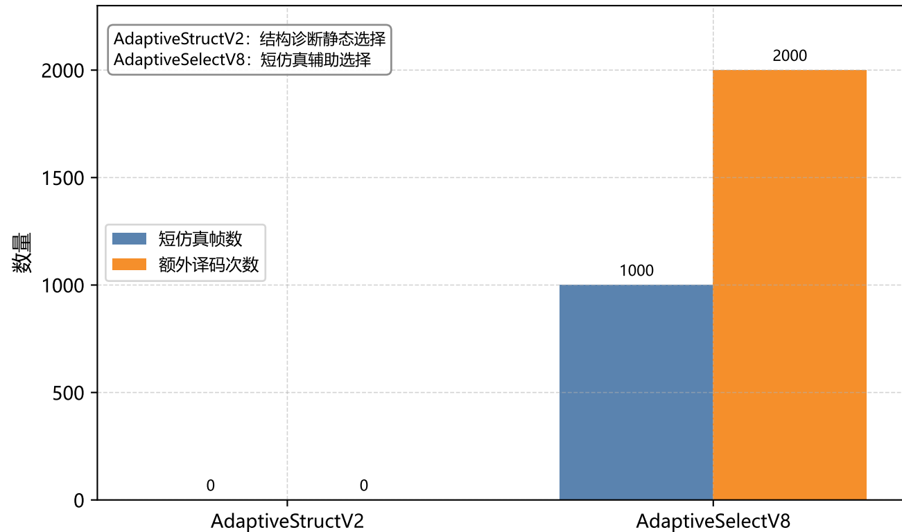
选择阶段开销对比
