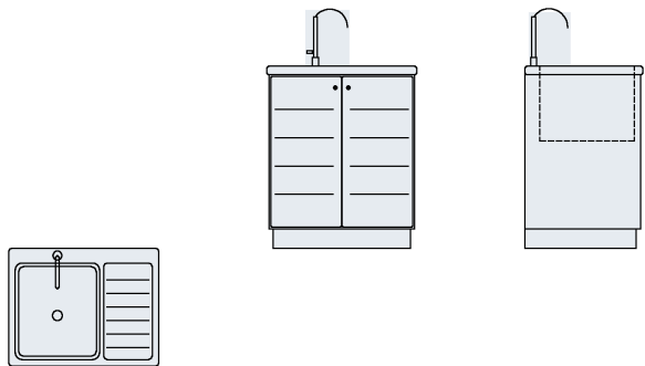
Chậu giặt 3 hình chiếu Rộng 700 Sâu 550 Cao 850
