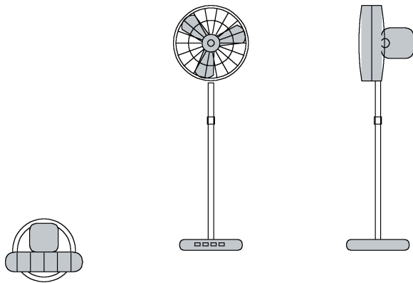
Quạt đứng 3 hình chiếu
