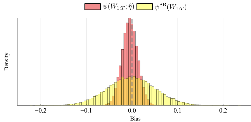
Hình 8: Hình 5 — So sánh DML4SSI với Switchback Horvitz-Thompson (SB). Cả hai đều không chệch nhưng DML4SSI có phương sai thấp hơn đáng kể (phân phối nhọn hơn).
