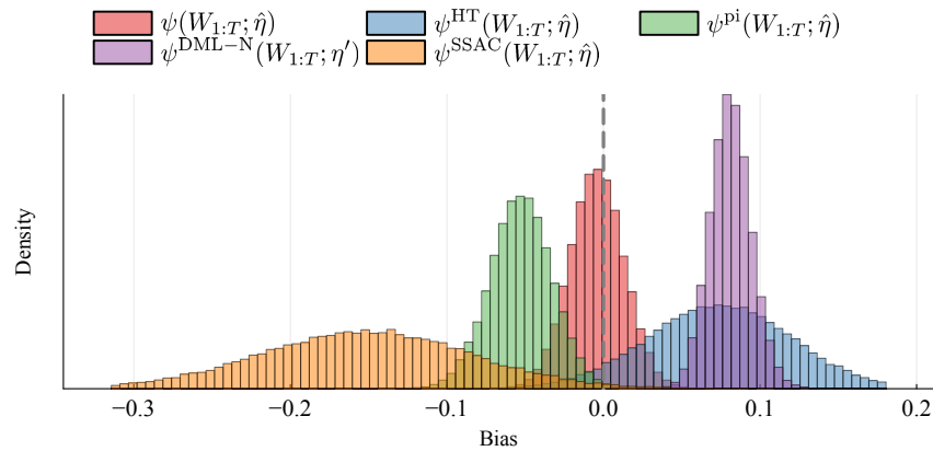
Hình 7: Hình 4 — Phân phối ước lượng điểm của GATE trong Switchback: DML4SSI so với các phương pháp naive. Các phương pháp naive bị chệch nặng; DML4SSI tập trung xung quanh giá trị thực.
