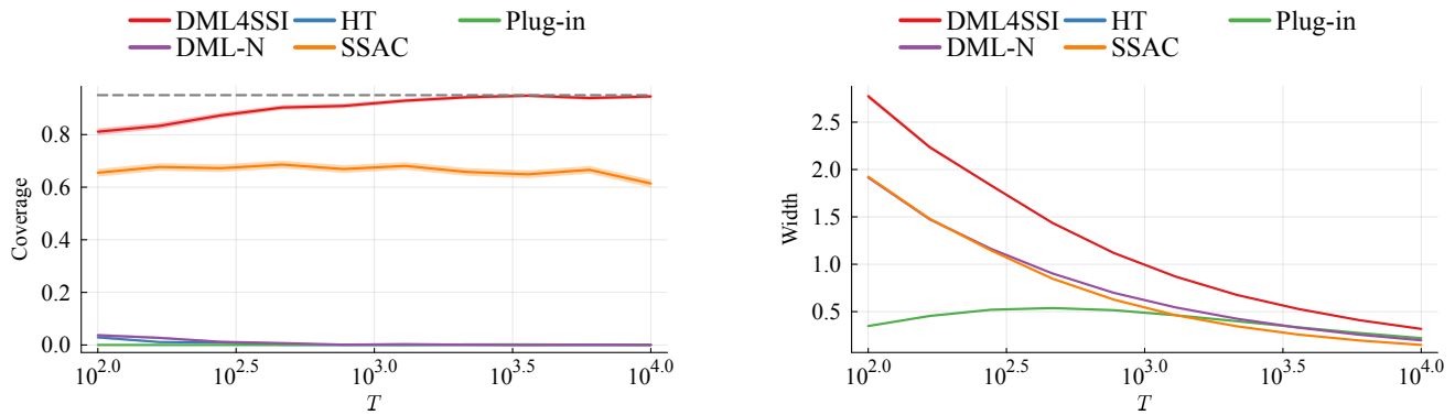
Hình 6: Hình 3 — Độ phủ (trái) và Độ rộng (phải) của khoảng tin cậy 95% cho ADE theo cỡ mẫu T . Chỉ DML4SSI hội tụ đến mức phủ chuẩn 95%; SSAC bị kẹt ở 60–70% do đánh giá thấp phương sai.
