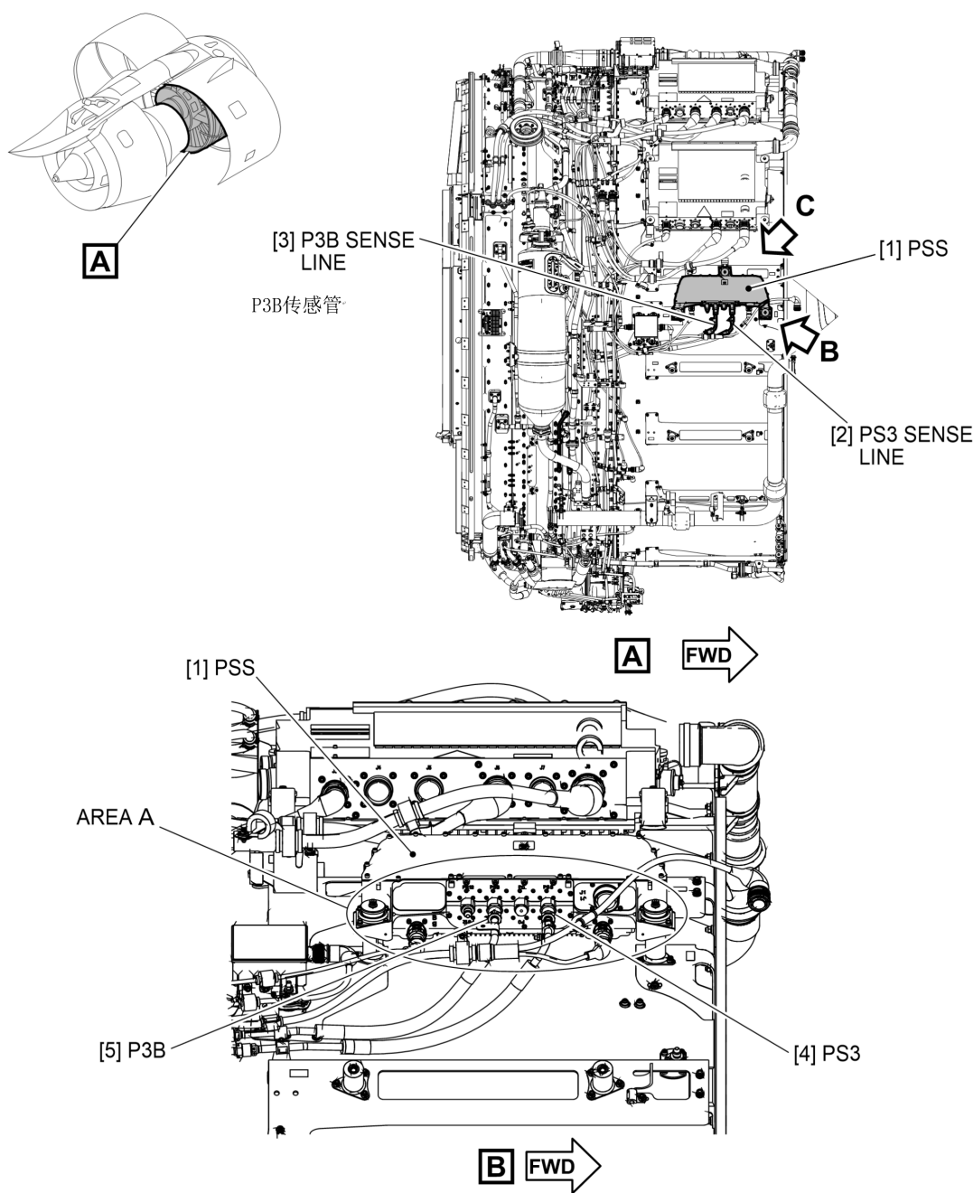
ICN-C919-A-732145-B-58828-07000-A-002-01 (1/2) PSS , PS3 sense line, and P3B sense line 图1 PSS、PS3传感管和P3B传感管(共2张第1张) ON A/C MSN ALL
