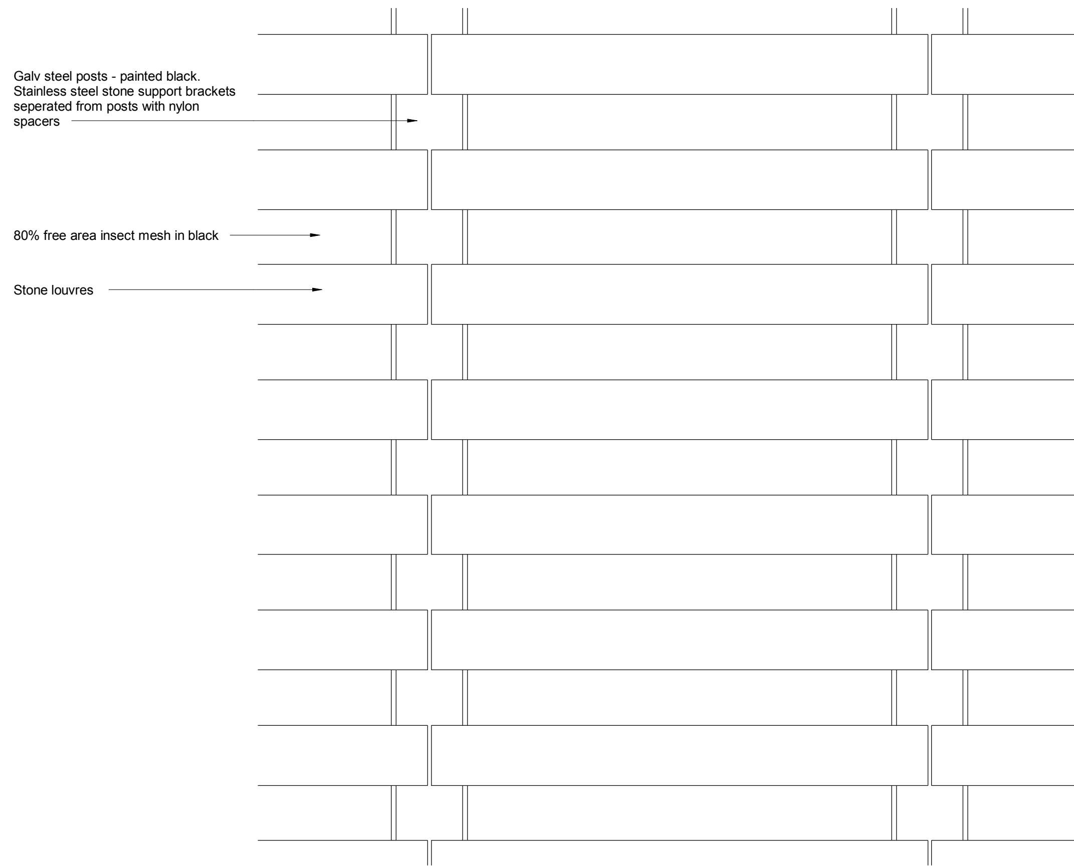
2 580-23 - Elevation 1:5
