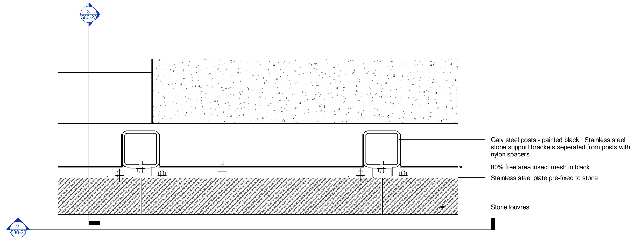
1 580-23 - Plan 1:5
