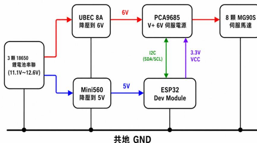
四足機器狗簡化接線方塊圖
