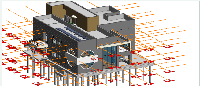
실제 BIM 모델 (Revit)
