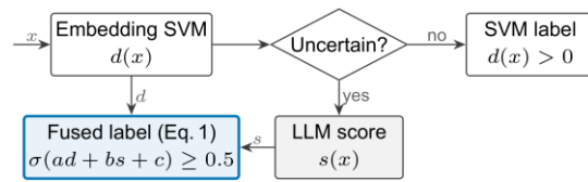
그림 1. 결합형 캐스케이드의 구조
