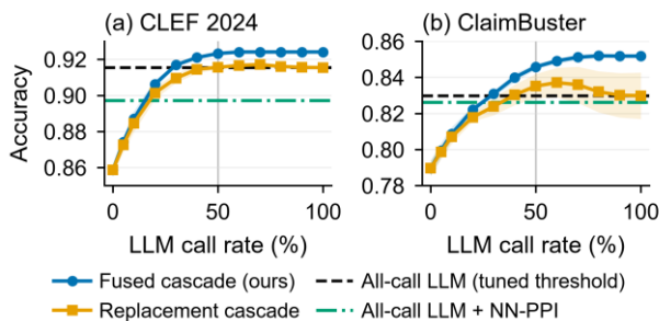
그림 2. 호출률에 따른 테스트 정확도 (5회 평균, 떠는 표준편차)
