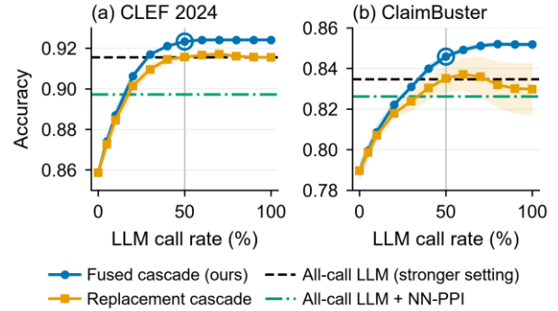
그림 2. 결합형은 호출률 50%(원)에서 이미 LLM 전량 호출(점선)에 도달한다. 5회 평균, 띠는 표준편차. 점선은 LLM 전량 호출 중 더 나은 설정(CLEF는 임계값 조정, ClaimBuster는 조정 전)이다.
