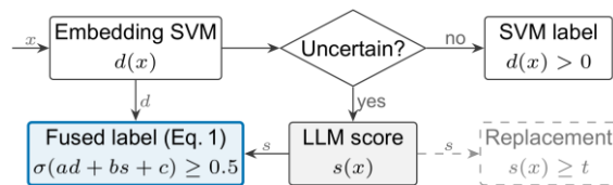
그림 1. 결합형 캐스케이드의 구조. 분류기가 불확실한 문장에서만 LLM을 호출하고, LLM 점수 s 를 분류기 결정값 d 와 결합한다. 점수는 비교 대상인 교체형으로, d 를 버리고 s 만 임계값 t 와 비교한다.
