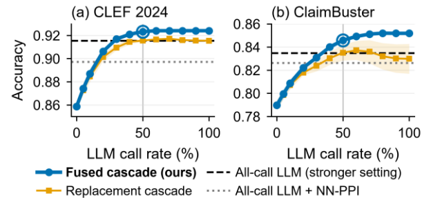
그림 2. 호출률에 따른 테스트 정확도 (5회 평균, 띠는 표준편차)
