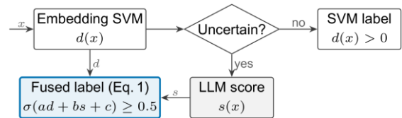
그림 1. 결합형 캐스케이드의 구조
