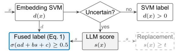
그림 1. 결합형 캐스케이드의 전체 구조
