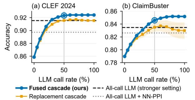
그림 2. 호출률에 따른 테스트 정확도 (5회 평균, 띄는 표준편차)
