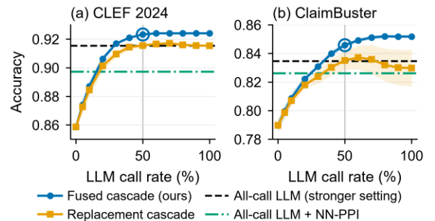
그림 2. 호출률에 따른 테스트 정확도 (5회 평균, 띠는 표준편차)
