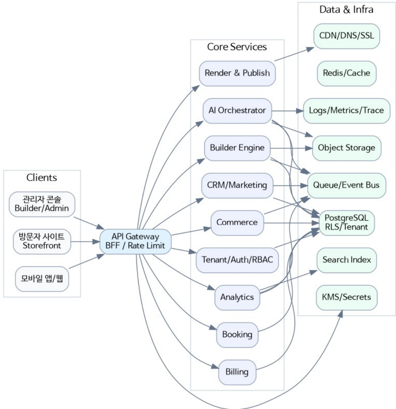
그림 2. WEBABLE SaaS 시스템 아키텍처 - 클라이언트, 코어 서비스, 데이터/인프라 계층을 분리한다.
