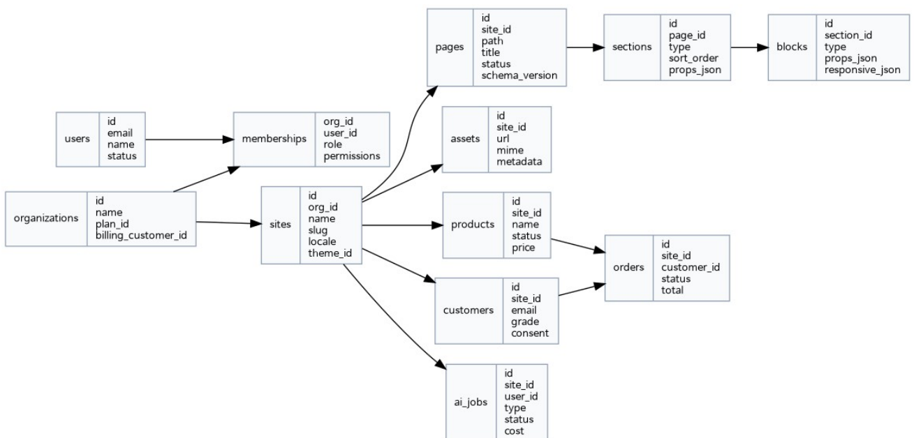
그림 3. 고수준 ERD - 조직, 사이트, 페이지, 섹션/블록, 커머스, 고객, AI 작업을 중심으로 구성한다.
