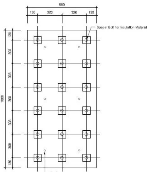
A. Spacer Bolt
