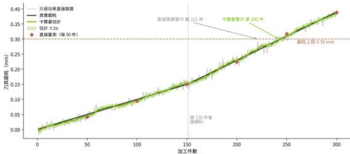
圖 19-7 以卡爾曼濾波器估計刀具磨耗與剩餘壽命
