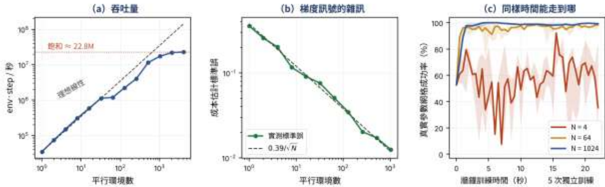
圖 33-1 平行環境數的三個效果：吞吐量、梯度雜訊與訓練穩定度
