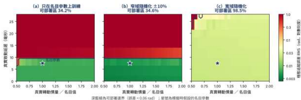
圖 33-4 域隨機化的範圍對部署成功率的影響
