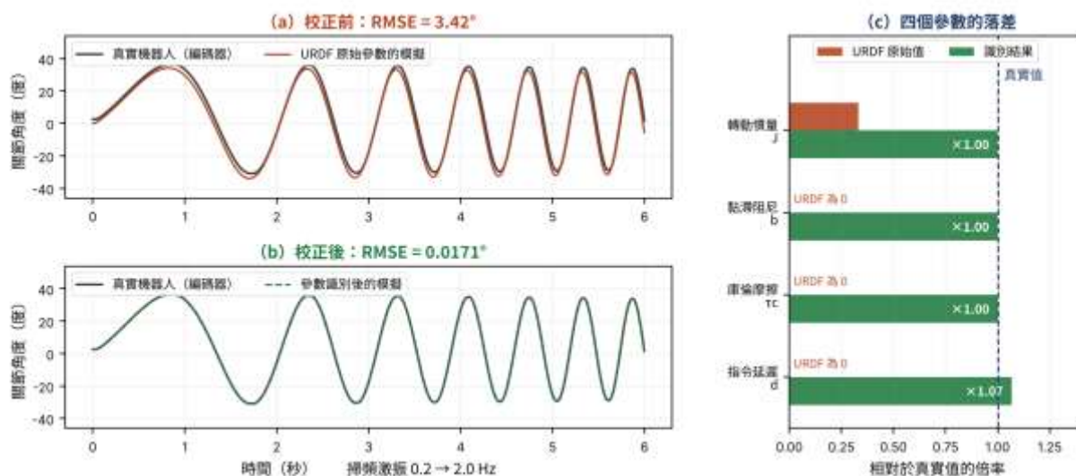
圖 33-3 系統識別：從 URDF 的猜測到擬合後的模擬
