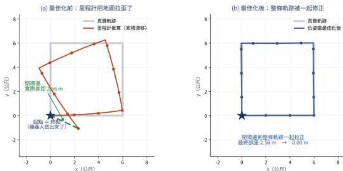
圖 12-2 閉環的威力：一條邊如何把整張地圖拉正
