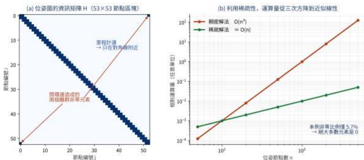
圖 12-3 稀疏性：上萬個節點也能即時求解的祕密
