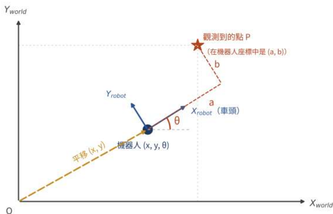
圖 10-1 2D 剛體變換：把機器人座標中的點搬到世界座標
