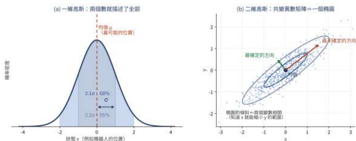
圖 11-1 高斯分布：從一維鐘形曲線到二維不確定性橢圓
