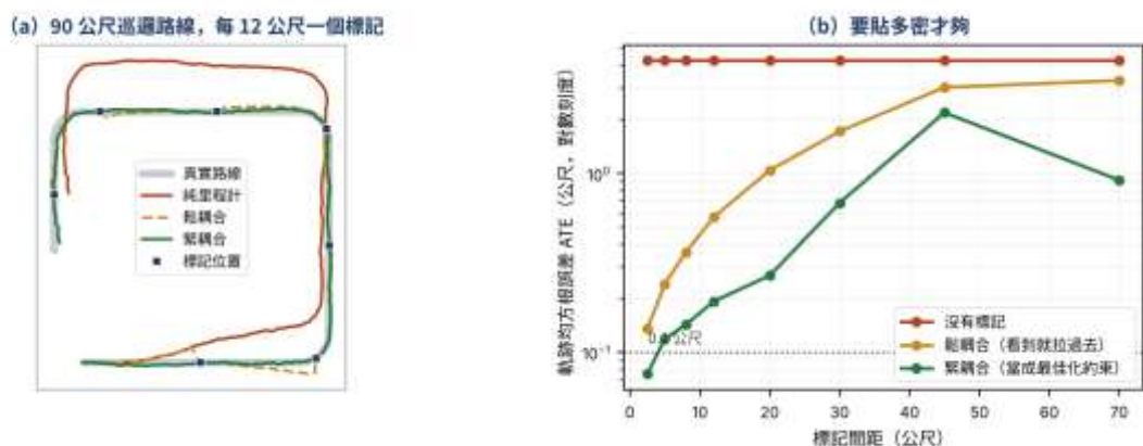
圖 24-3 標記間距對定位精度的影響
