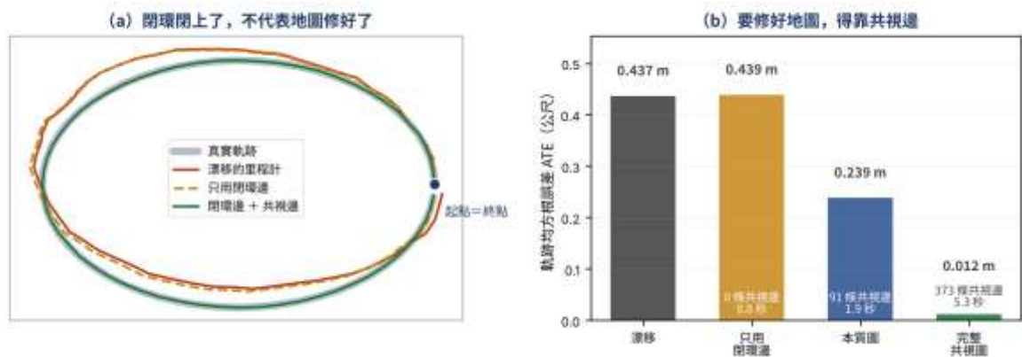
圖 22-2 閉環閉上了，不代表地圖修好了
