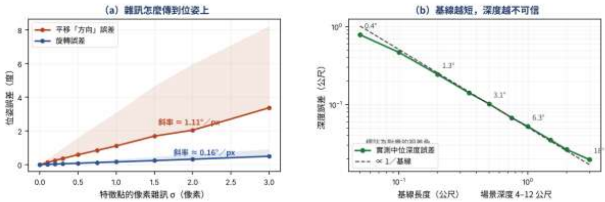
圖 21-3 雜訊如何傳到位姿，以及基線如何決定深度精度
