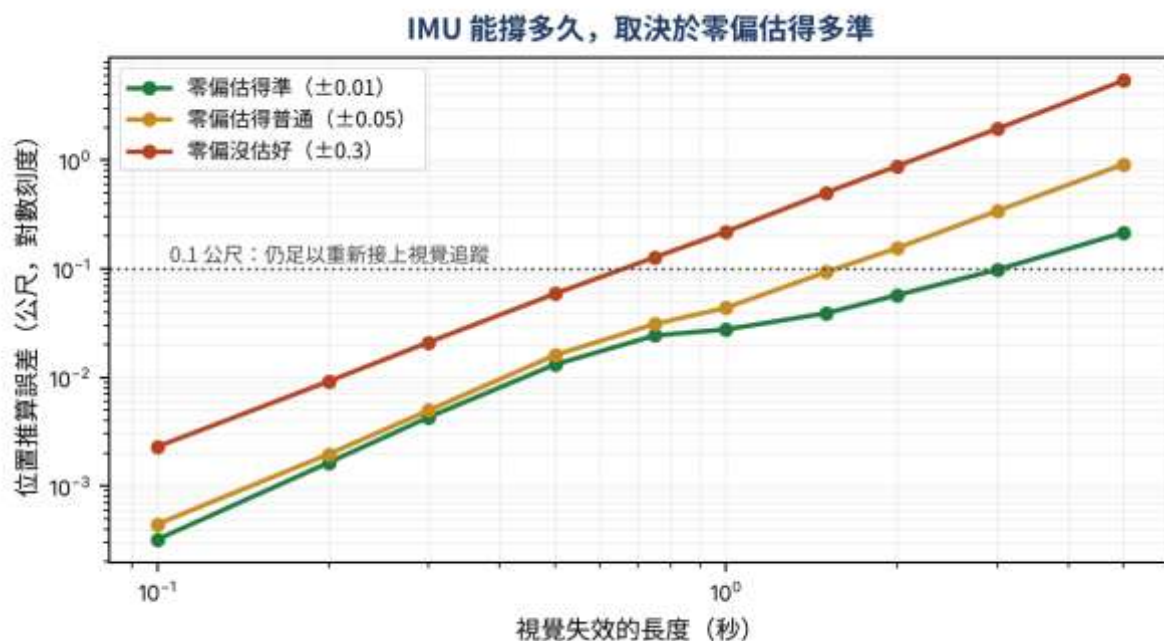
圖 23-1 IMU 能撐多久，取決於零偏估得多準
