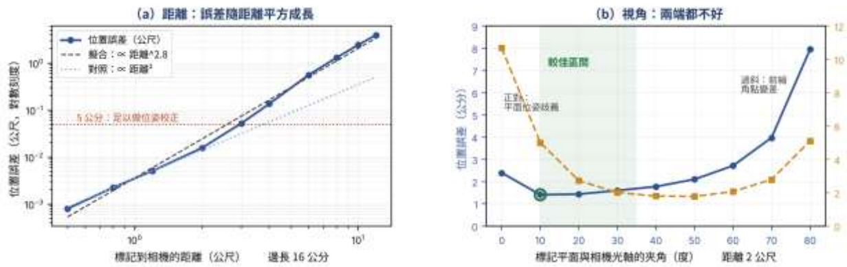
圖 24-2 標記的位姿精度如何隨距離與視角變化
