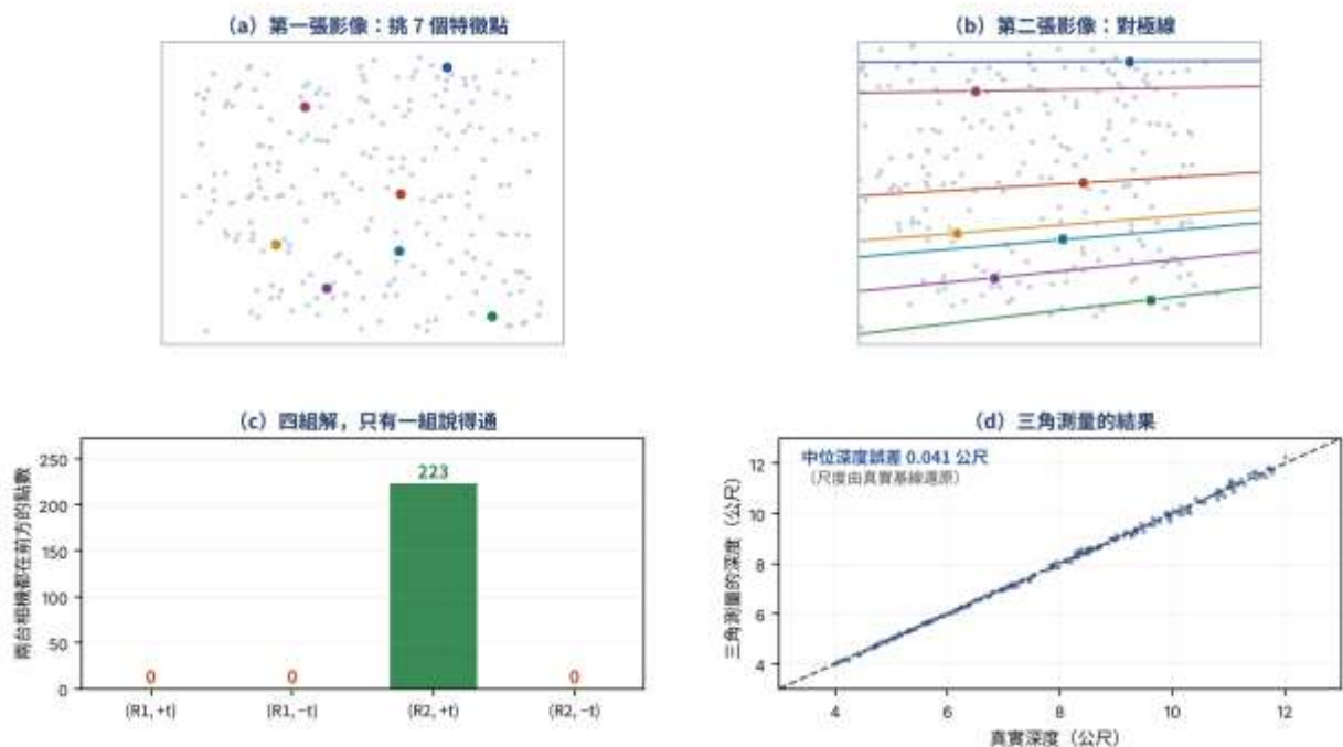
圖 21-2 對極約束的數值驗證：從對應點到三維座標
