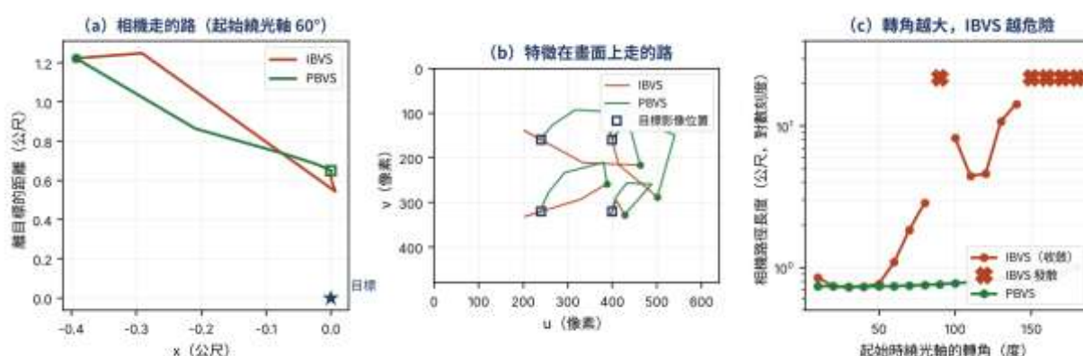
圖 24-1 影像式與位置式視覺伺服的收斂行為
