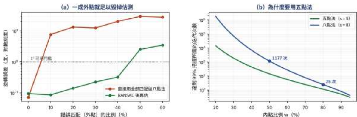
圖 21-4 誤匹配的代價，以及取樣點數為何關鍵
