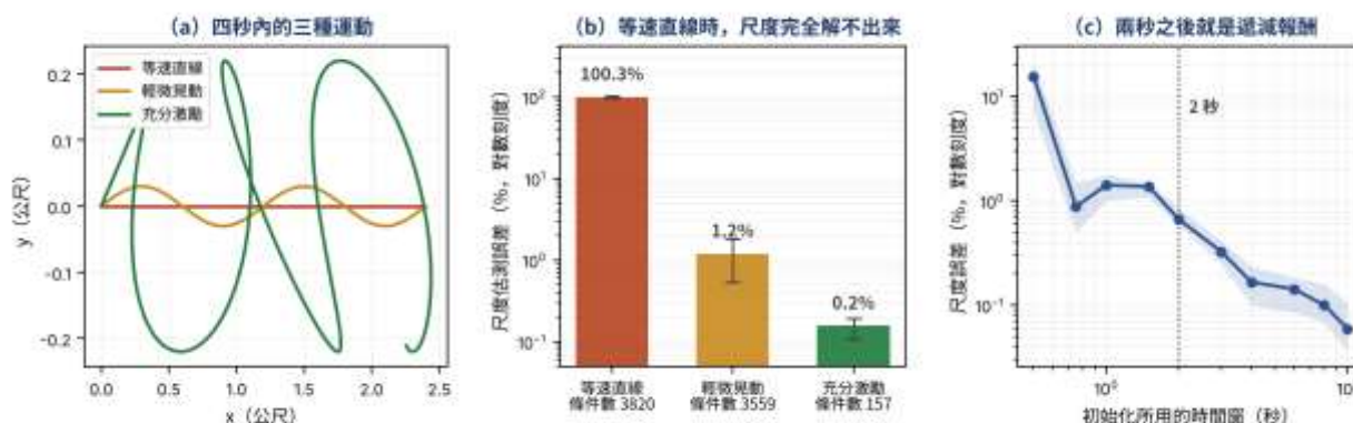
圖 23-2 運動激勵決定了初始化能不能解
