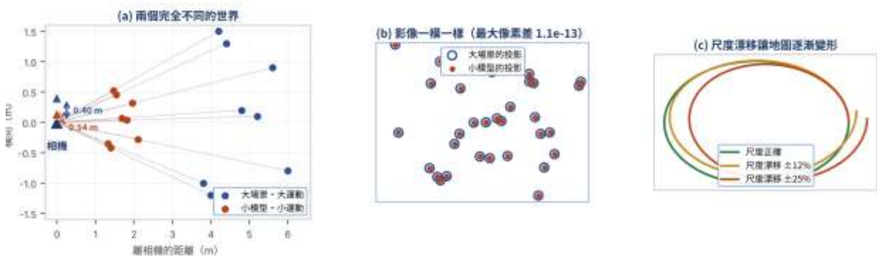
圖 20-4 尺度不確定性：單目相機先天無法分辨的兩個世界
