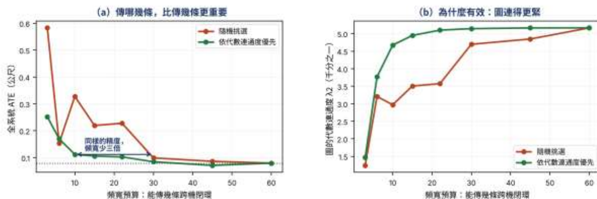
圖 27-3 有限頻寬下，該優先傳哪些閉環候選
