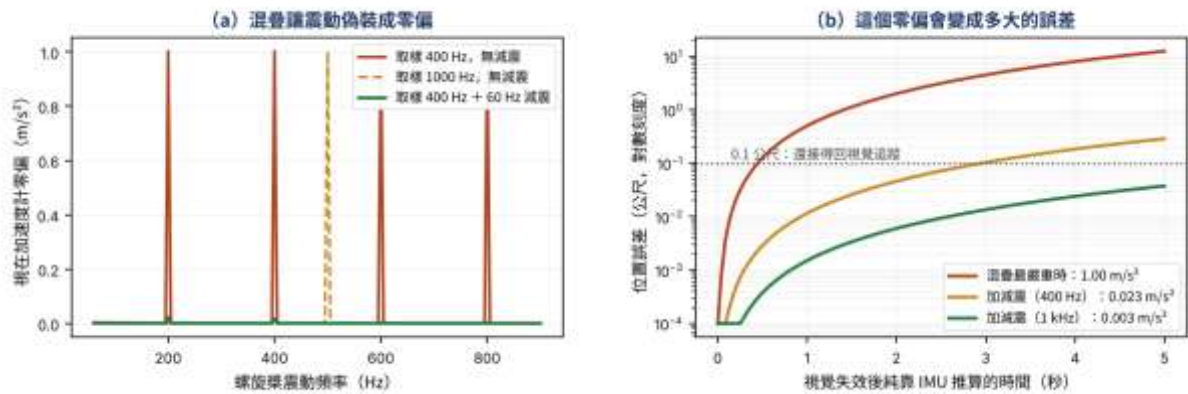
圖 26-3 震動的混疊，以及它為什麼偽裝成零偏
