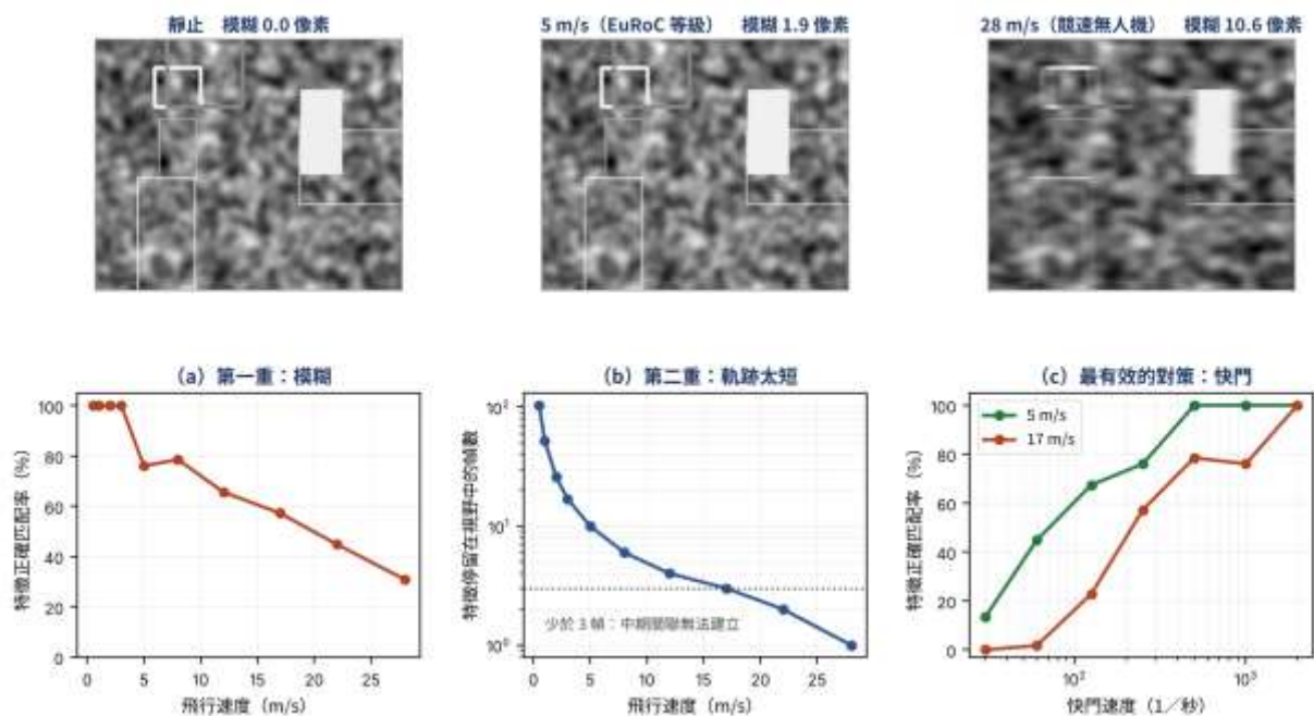
圖 26-2 速度造成的三重打擊，以及最有效的對策
