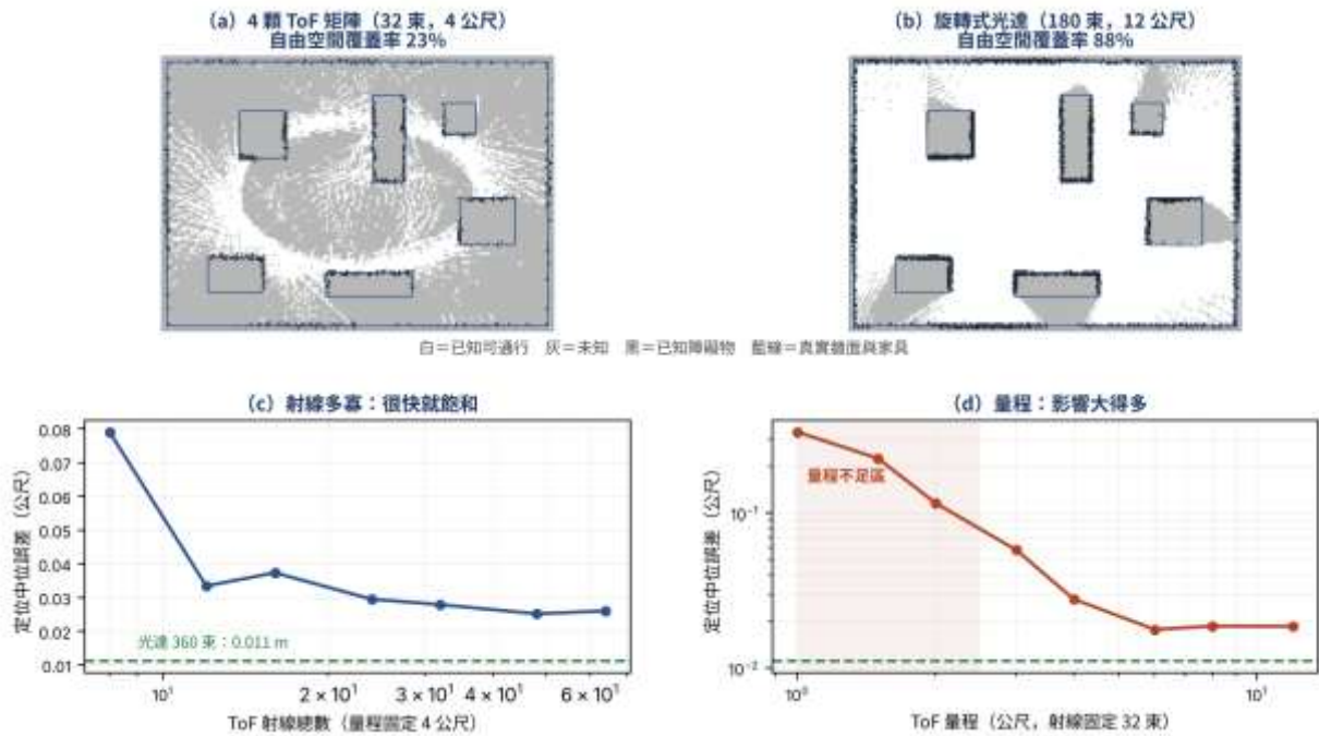
圖 25-3 稀疏 ToF 與旋轉式光達的建圖與定位
