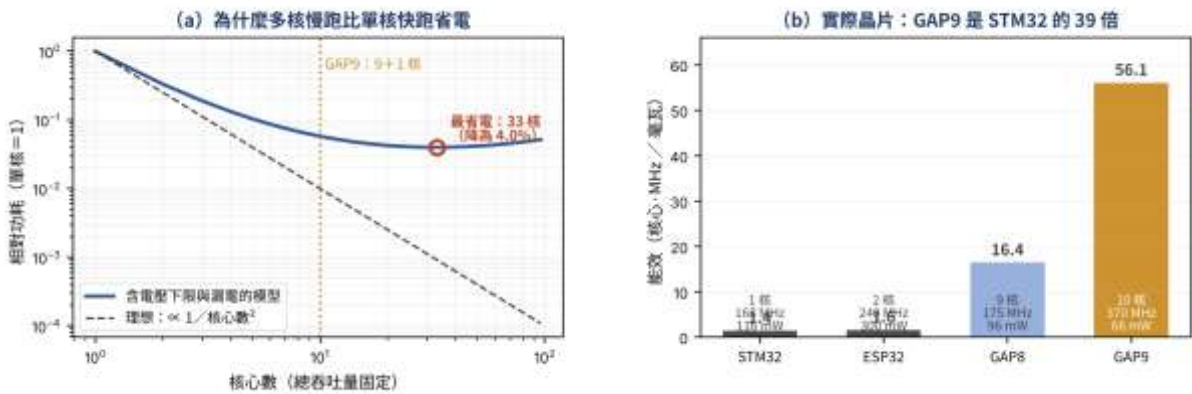
圖 25-1 PULP 的能效原理與實際晶片的對照
