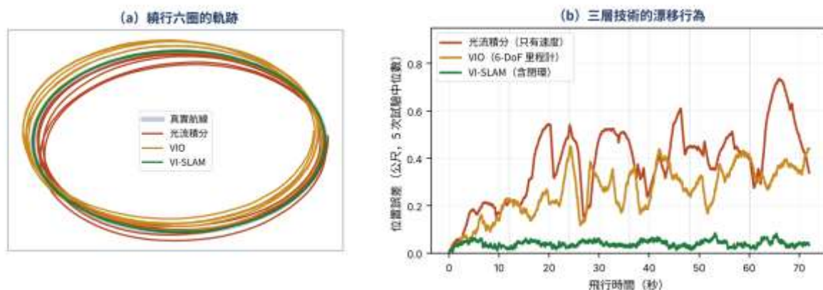
圖 26-1 光流、VIO 與 VI-SLAM 的漂移行為
