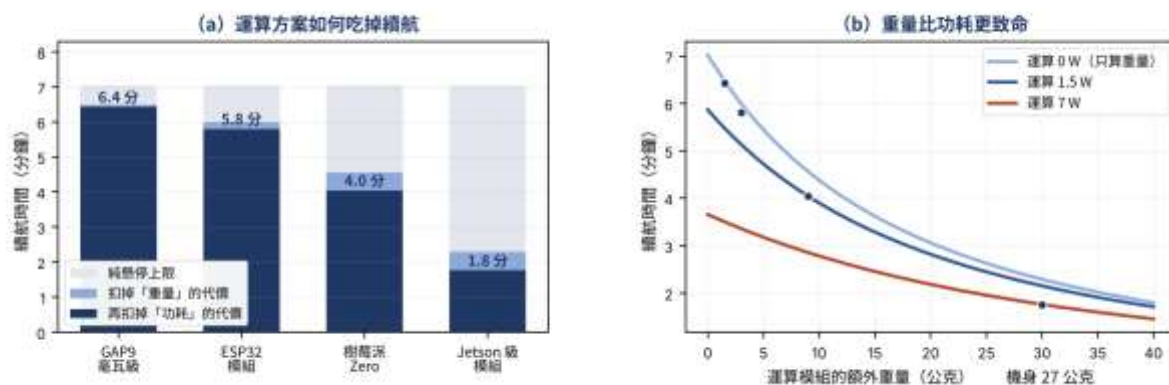
圖 25-4 運算方案的重量與功耗如何吃掉續航
