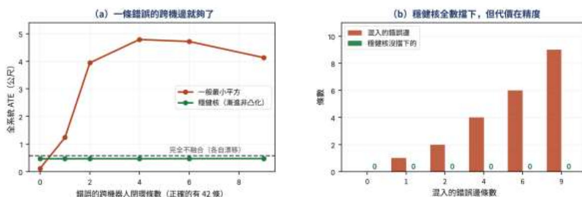
圖 27-2 錯誤的跨機器人閉環與穩健剔除
