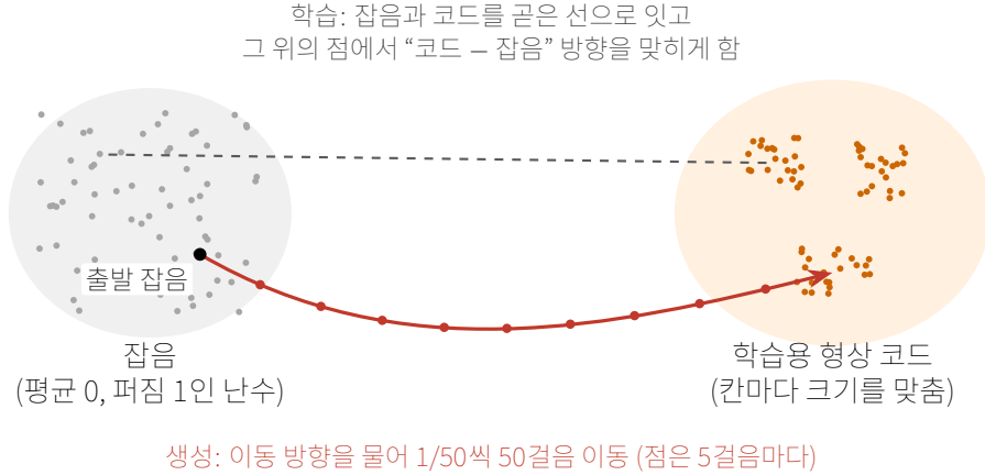
그림 10: 2단계 생성 모델이 하는 일. 학습 때는 잡음과 실제 코드를 곧은 선으로 이어 “가야 할 방향”을 가르친다(회색 점선). 생성 때는 새 잡음에서 출발해 매 걸음 방향을 물어 50걸음에 걸쳐 코드가 모인 곳으로 간다(빨간 선). 그림의 점 구름은 설명을 위한 가상 예시다.
