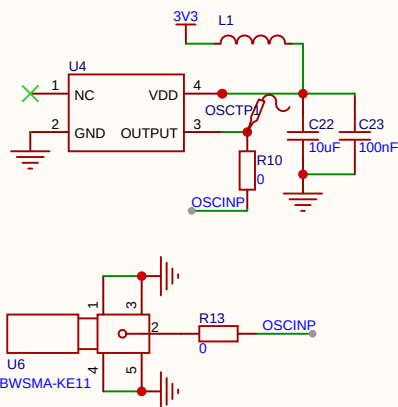
TXCO & 外部时钟参考
