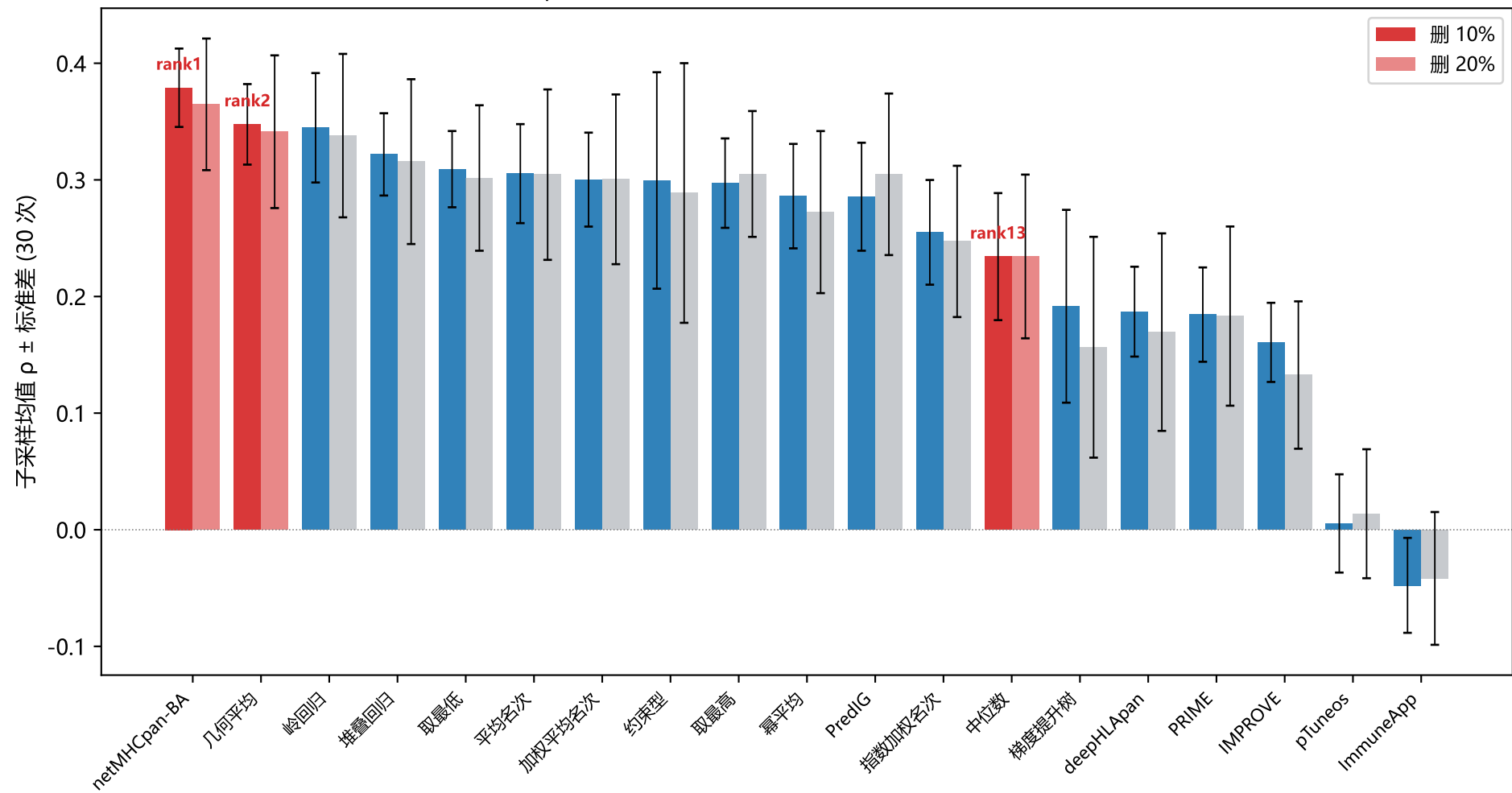
图 B | 随机删突变的稳健性 (固定窗口9肽 · 8位患者 · n=8) 红色高亮: netMHCpan-BA取最高(单工具) / 几何平均 / 中位数 (名次见标注, 按删10%排序)
