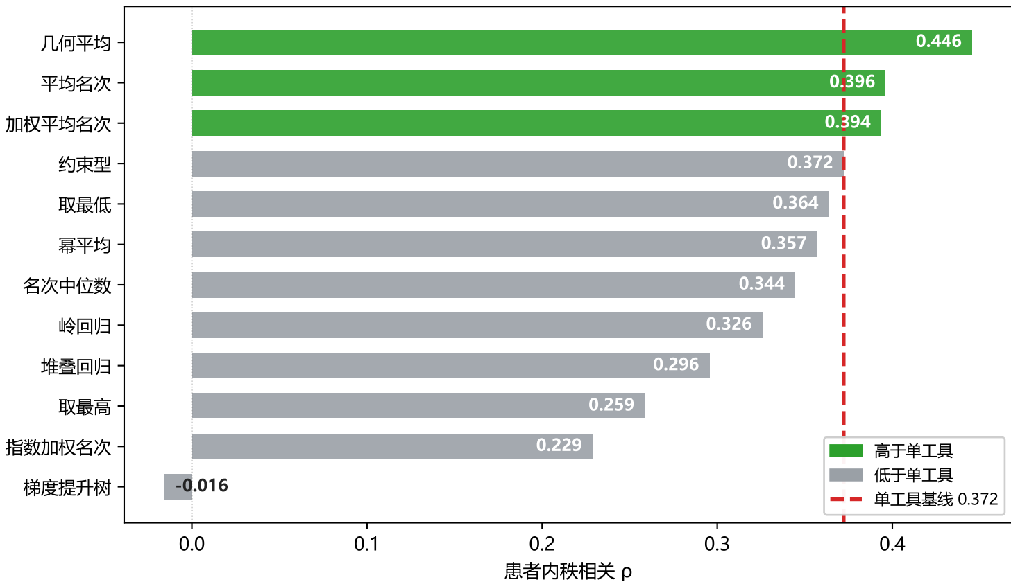
图 E | 三工具面板 (netMHCpan-BA+PRIME+deepHLApan) 各聚合函数 vs 最强单工具 (固定窗口9肽 · 8位患者 · n=8) 几何平均最高 (0.446); 3/12 个聚合函数高于单工具基线
