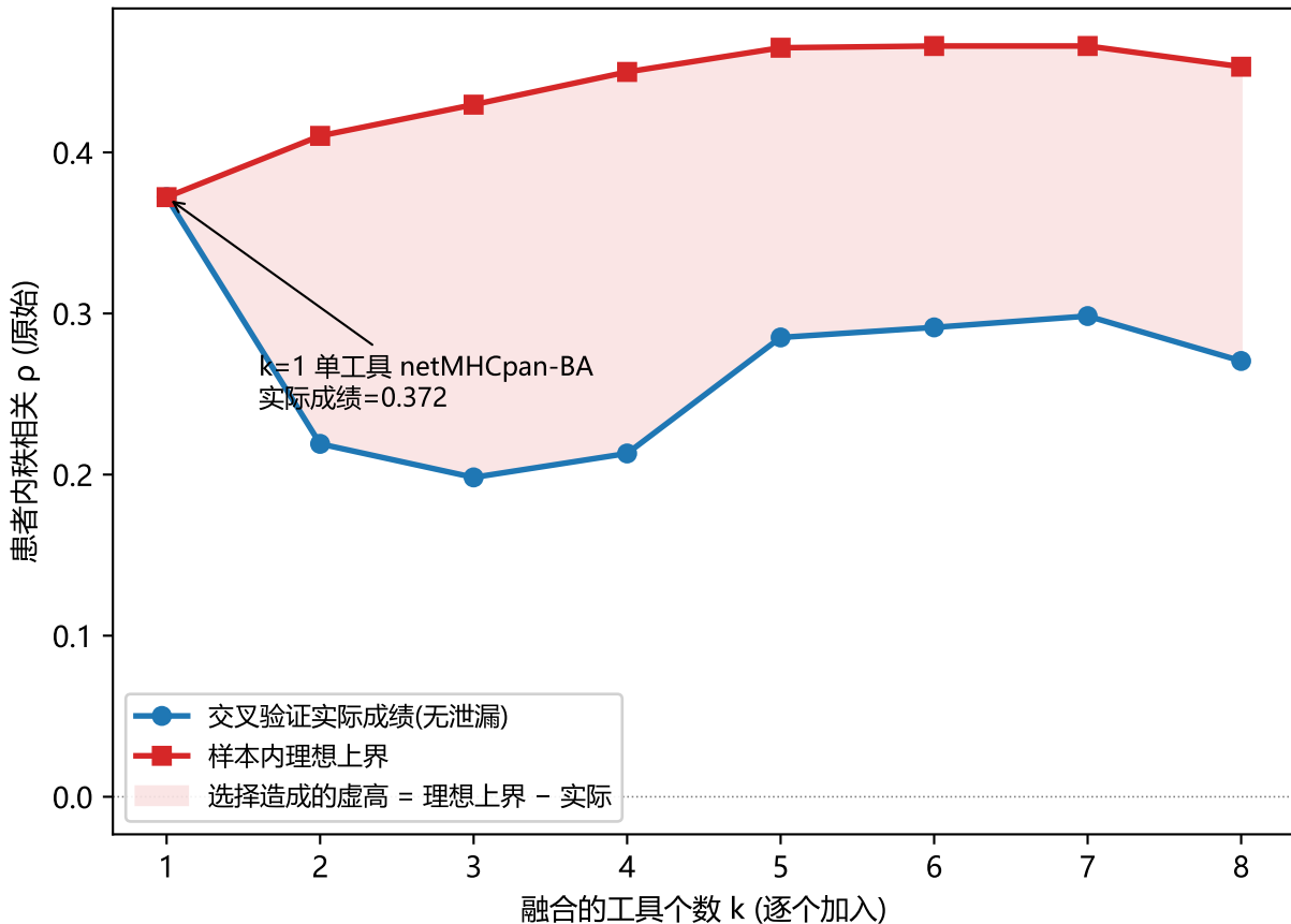
图 A | 融合工具个数 k 下 交叉验证实际 vs 样本内理想 (固定窗口9肽 · 8位患者 · n=8 ) 融合 \geq 2 个工具 对最强单工具 配对 p 最小 = 0.12 (均 > 0.05 )
