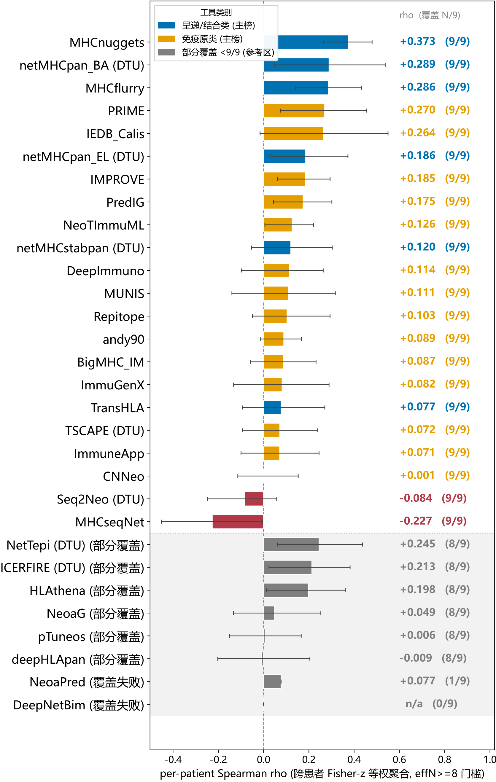
30 工具 per-patient Spearman (8-11mer 口径; 主榜=9/9 全覆盖工具, effN>=8 门槛)
