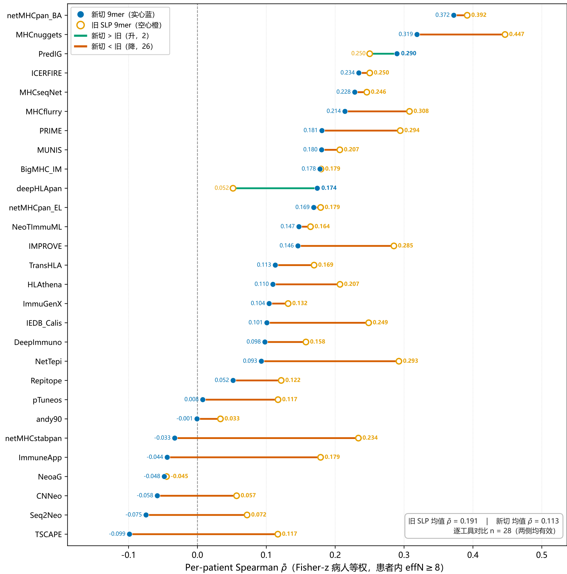
9mer 新切肽 vs 旧 SLP 切肽：改动②去肽长混杂后单工具排序能力变化
