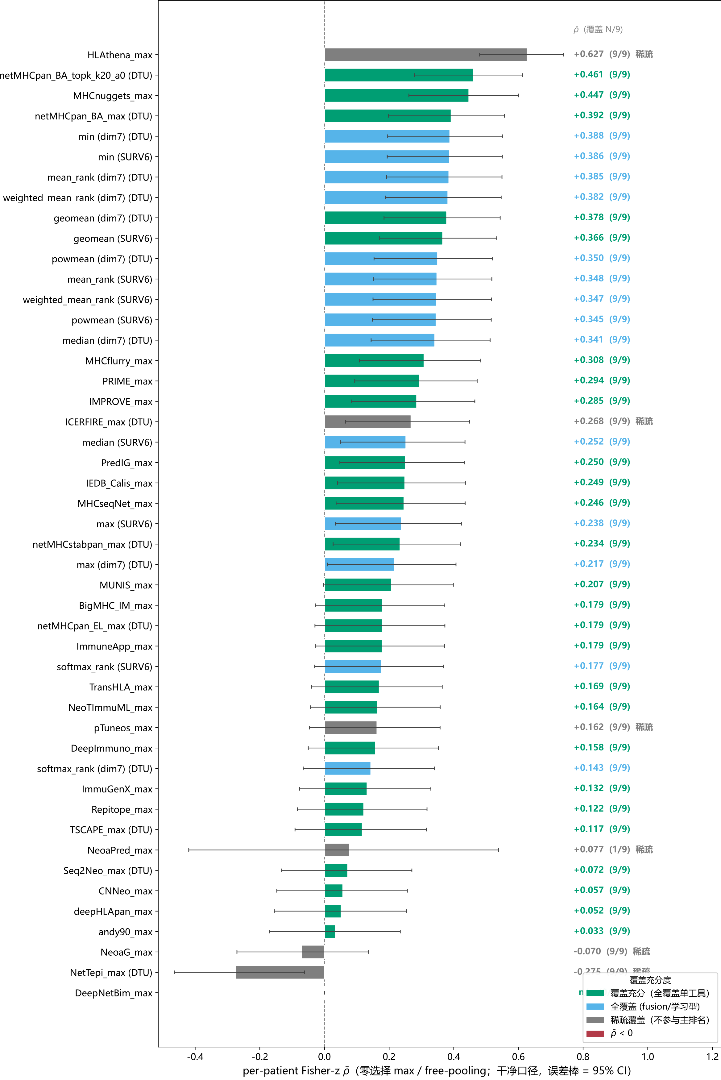
图4 · 全方法统一 LOPO 排名 (DS2 9 患者, 干净 canonical)
