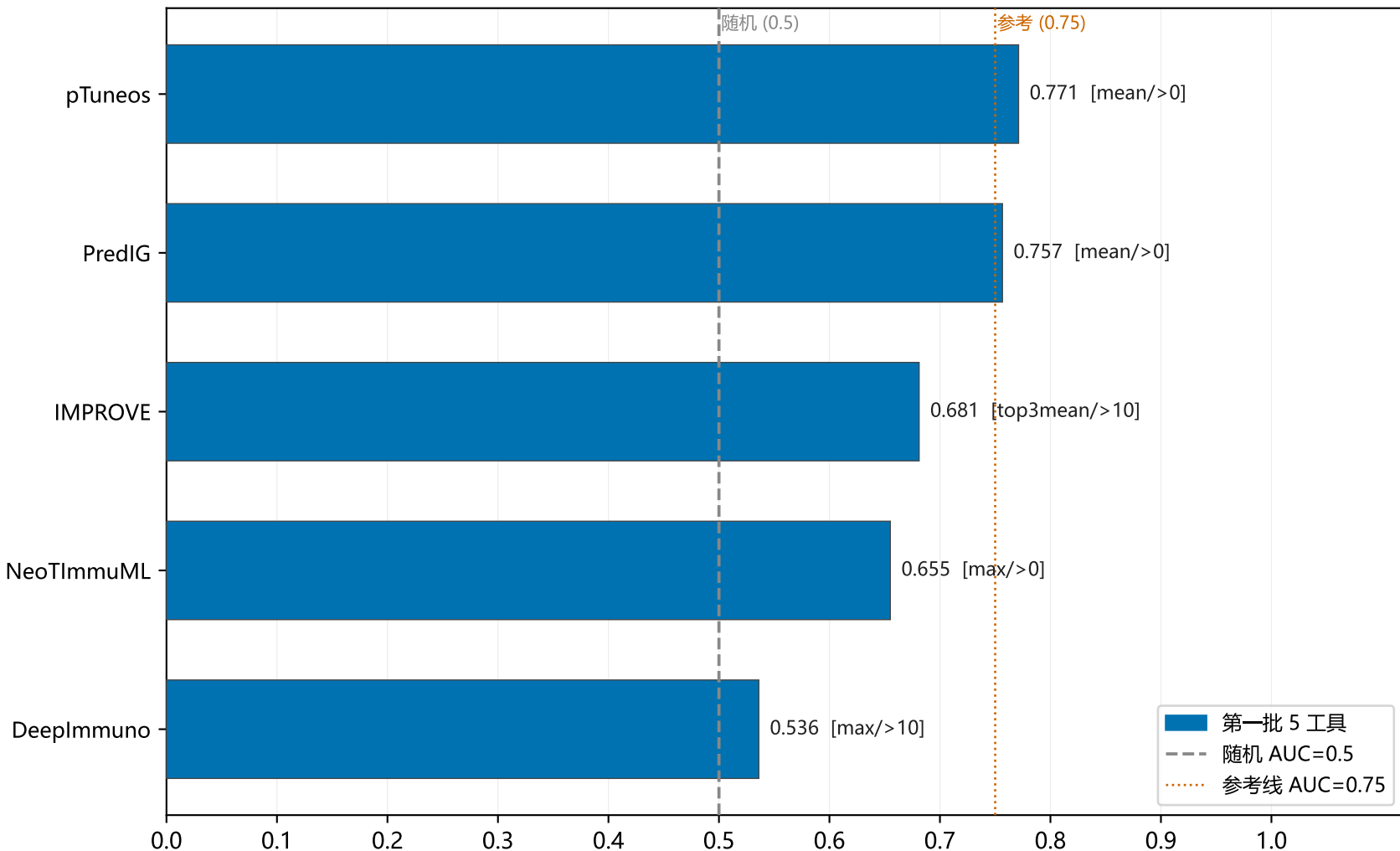
第一批 5 工具 AUC-ROC — DS2 HLA 修正后 每工具取最高 AUC 的聚合方式与阈值组合
