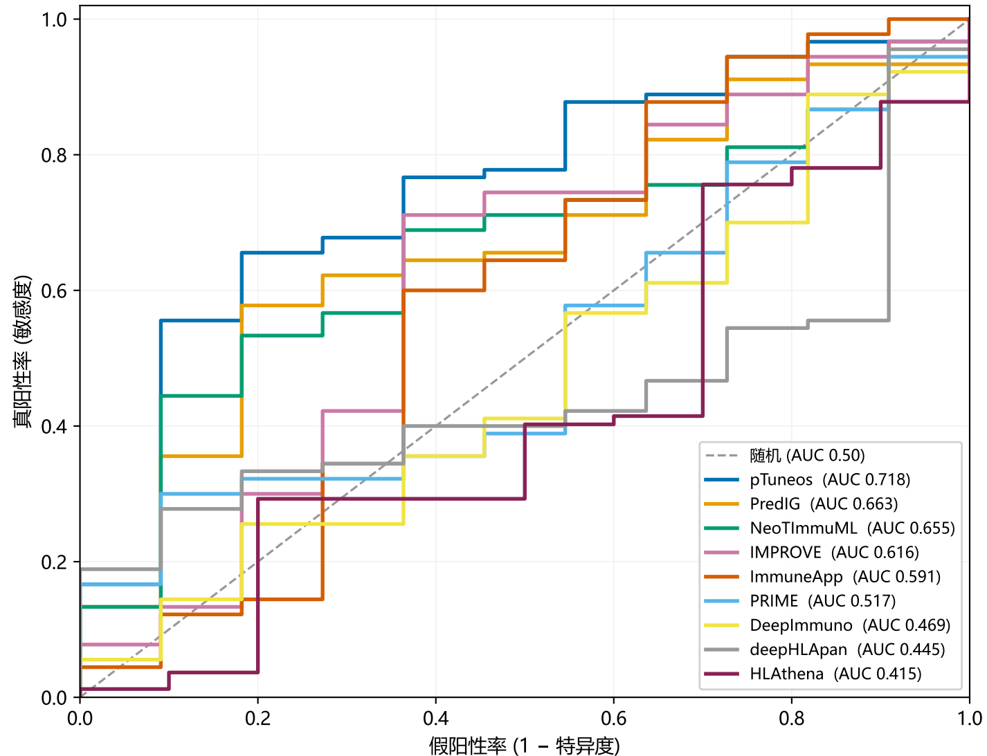
10 工具 ROC 曲线 — DS2 HLA 修正后 肽级最大分聚合, Elispot>0 为阳性; 曲线越凸向左上判别力越强
