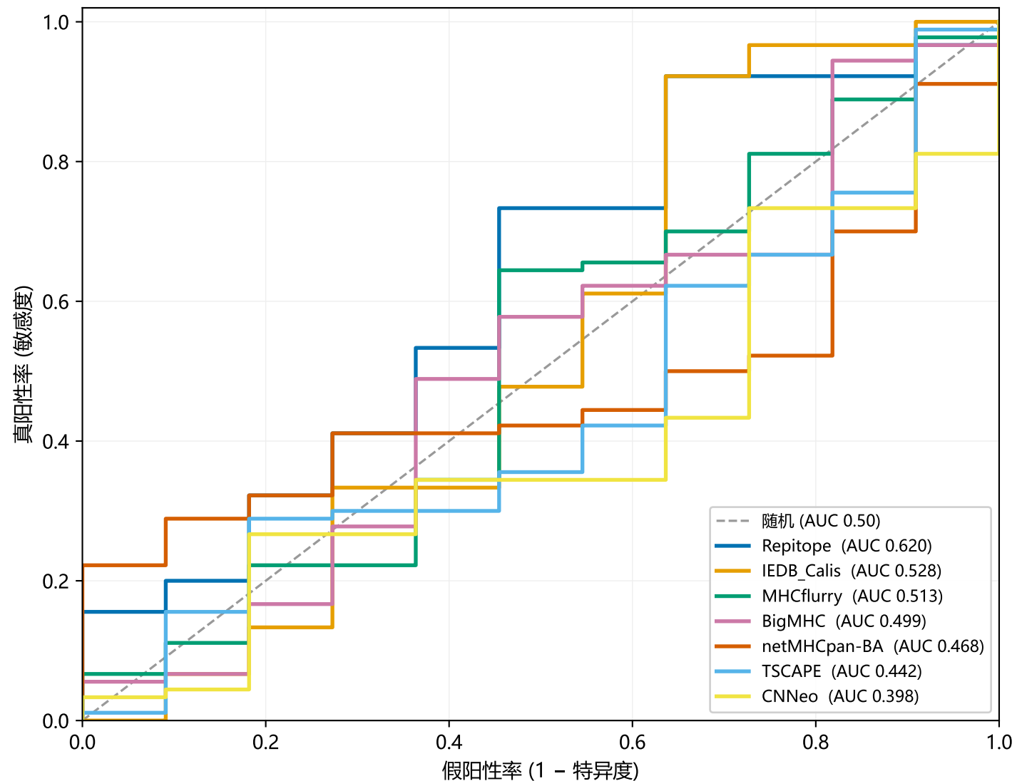
新增 7 工具 ROC 曲线 — DS2 HLA 修正后 肽级最大分聚合, Elispot>0 为阳性; 曲线越凸向左上判别力越强
