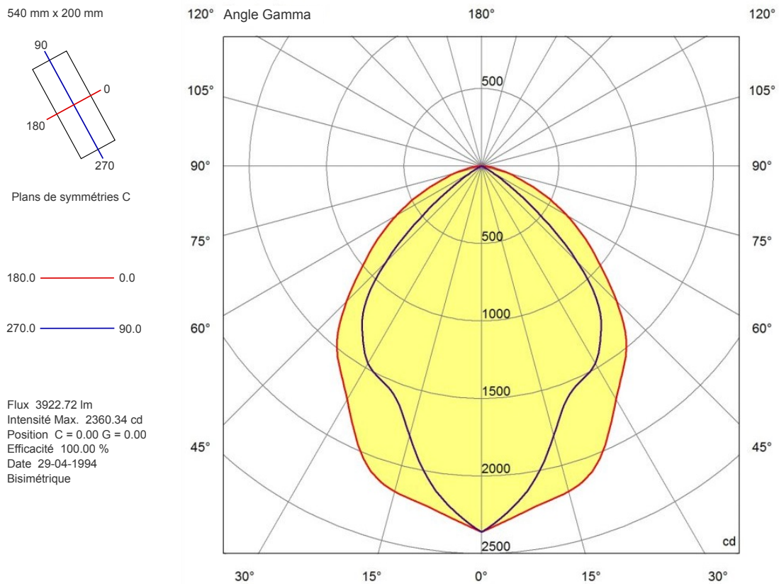
Figure 2: Fiche technique du luminaire utilisé. L'indicatrice d'intensité (droite) est donnée pour ses plans de symétrie longitudinal ( C_{90}-C_{270} ) et transversal ( C_0-C_{180} ). Source: asselum.com.
