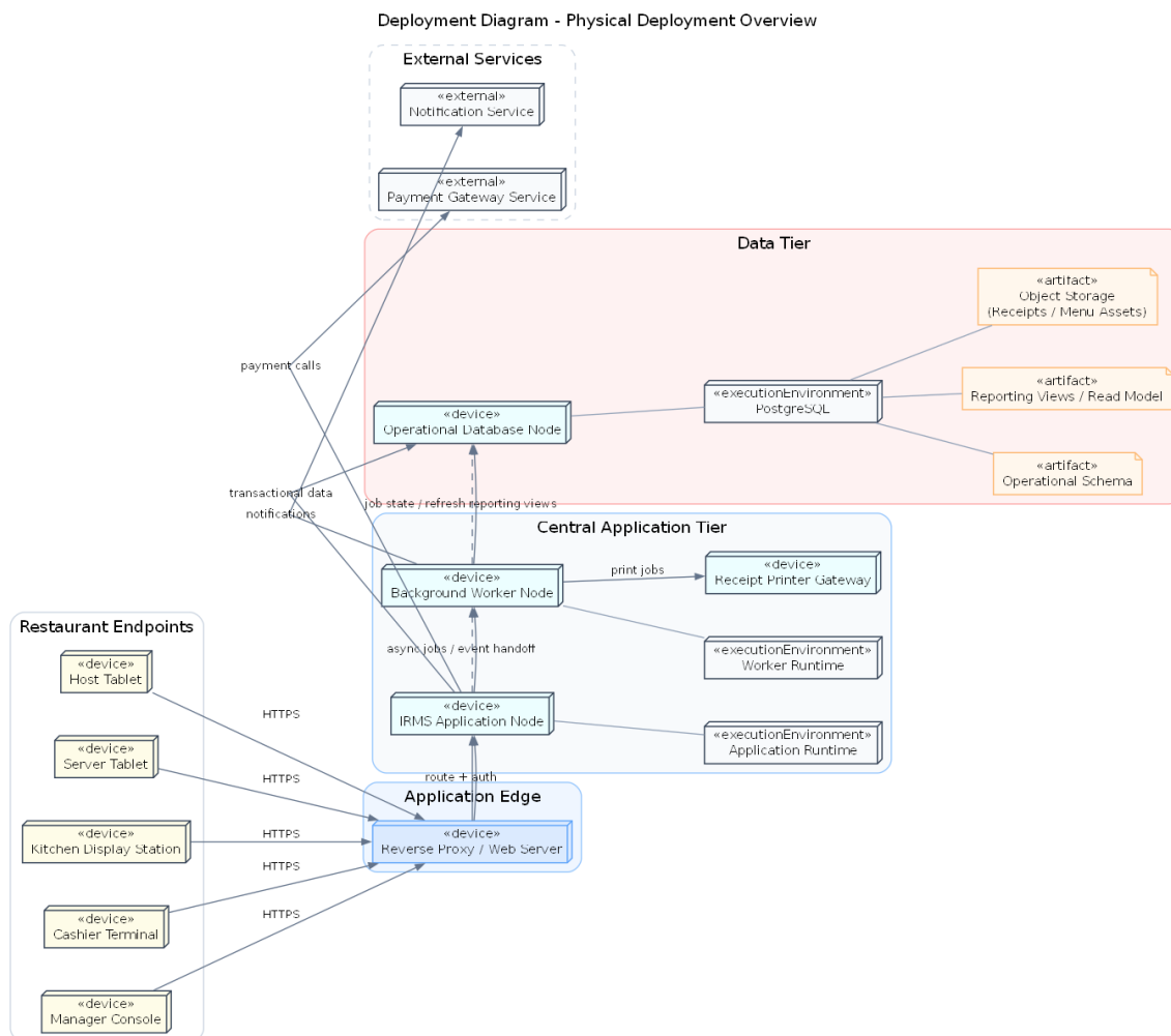
Hình 23: Sơ đồ triển khai tổng quan về bố trí vật lý của IRMS
