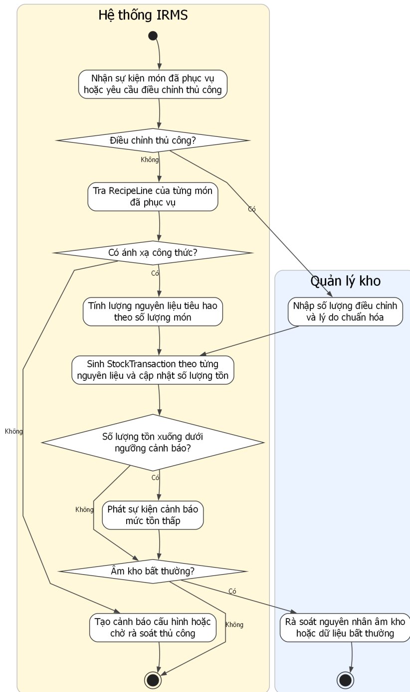
Hình 51: Sơ đồ hoạt động cho UC-INV-01 – Cập nhật tiêu hao tồn kho sau phục vụ
