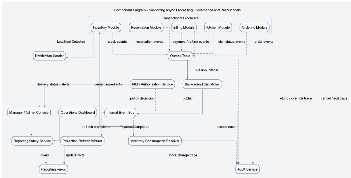
Hình 20: Sơ đồ thành phần cho xử lý nền, quản trị và mô hình đọc
