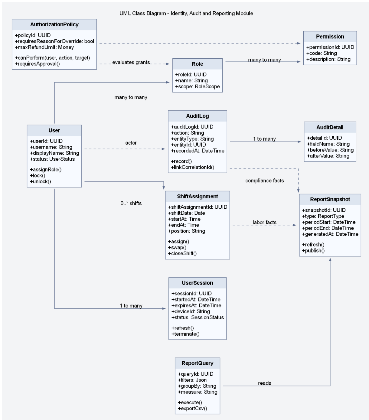
Hình 33: Sơ đồ lớp chi tiết cho module Identity, Audit &amp; Reporting
