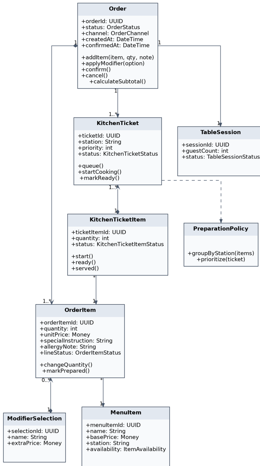
Hình 26: Sơ đồ lớp UML của cụm gọi món, thực đơn và bếp
