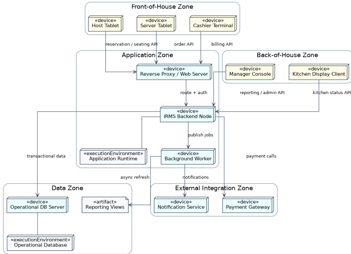
Hình 22: Sơ đồ triển khai theo vùng mạng và ranh giới tin cậy
