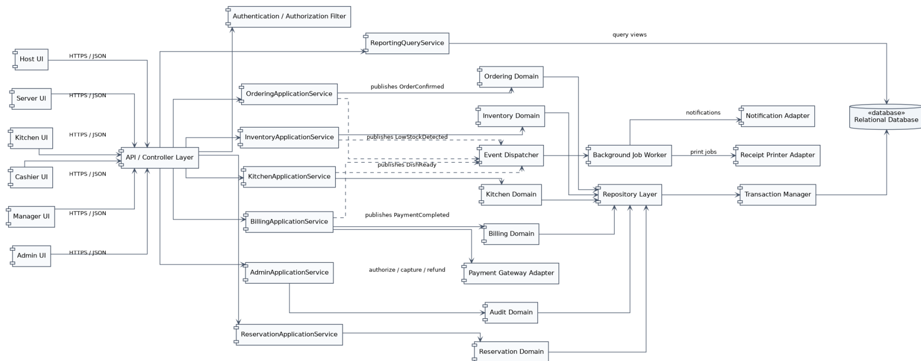
Hình 17: Sơ đồ thành phần và kết nối tổng quan của IRMS
