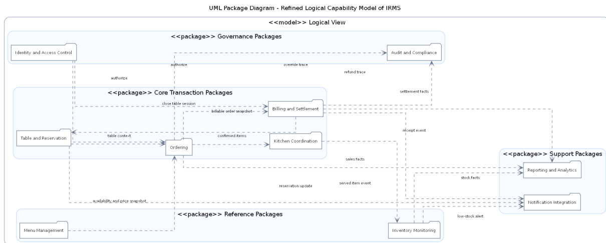
Hình 14: Sơ đồ phân rã năng lực logic của IRMS
