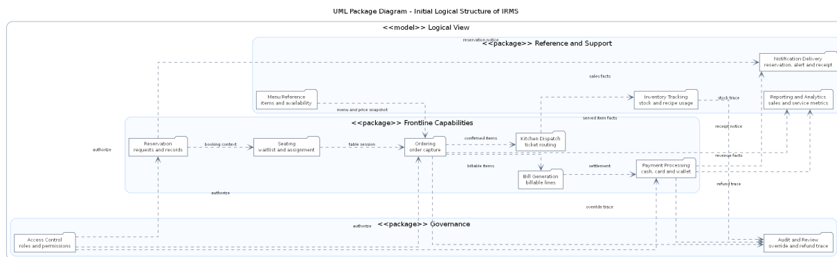
Hình 13: Sơ đồ phân rã năng lực logic ban đầu của IRMS
