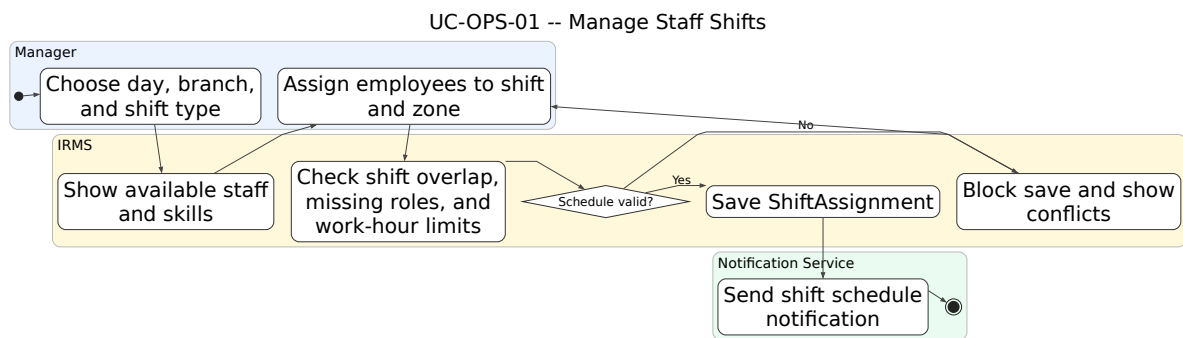
Hình 61: Sơ đồ hoạt động cho UC-OPS-01 – Quản lý ca làm nhân viên
