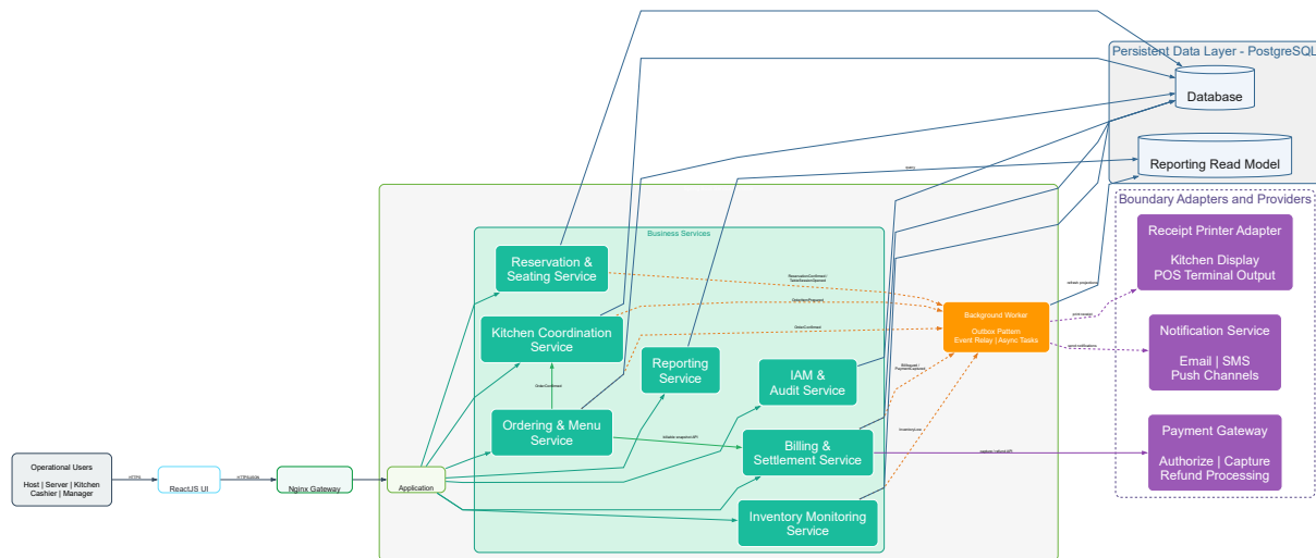
Hình 8: Sơ đồ tổng quan kiến trúc của IRMS
