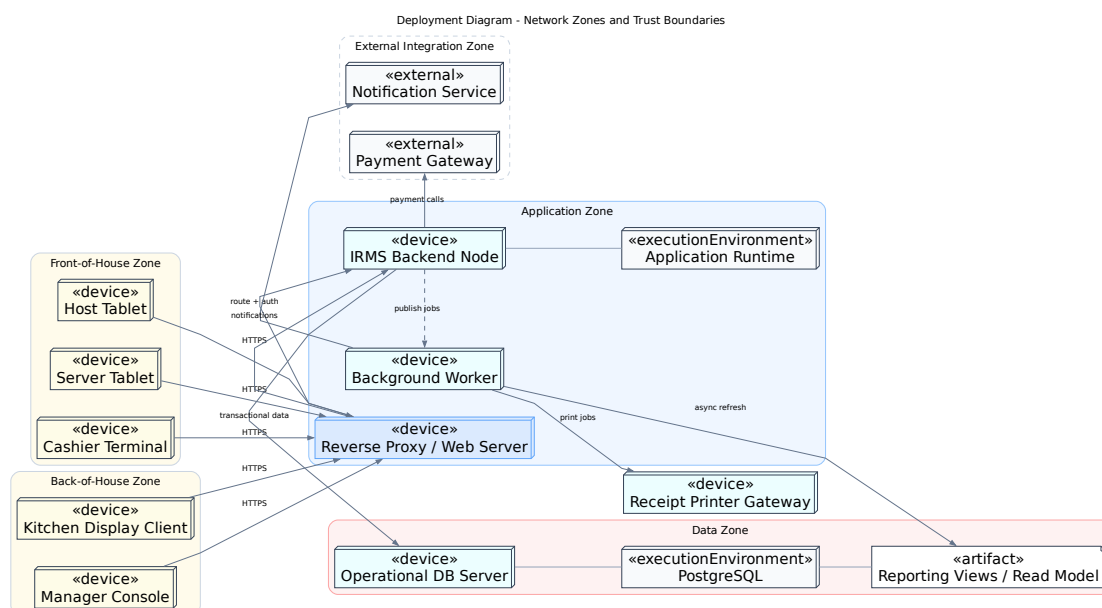
Hình 24: Sơ đồ triển khai theo vùng mạng và ranh giới tin cậy
