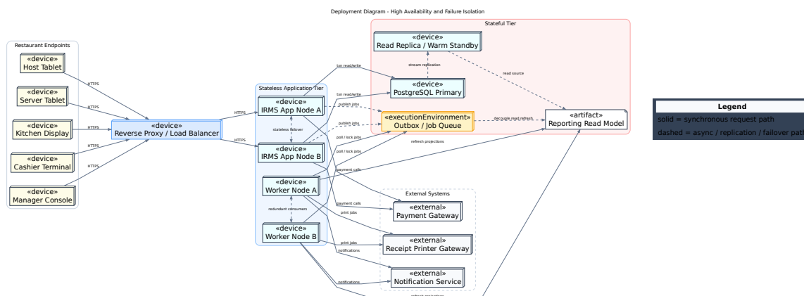
Hình 26: Sơ đồ triển khai cho tính sẵn sàng cao và cô lập lỗi
