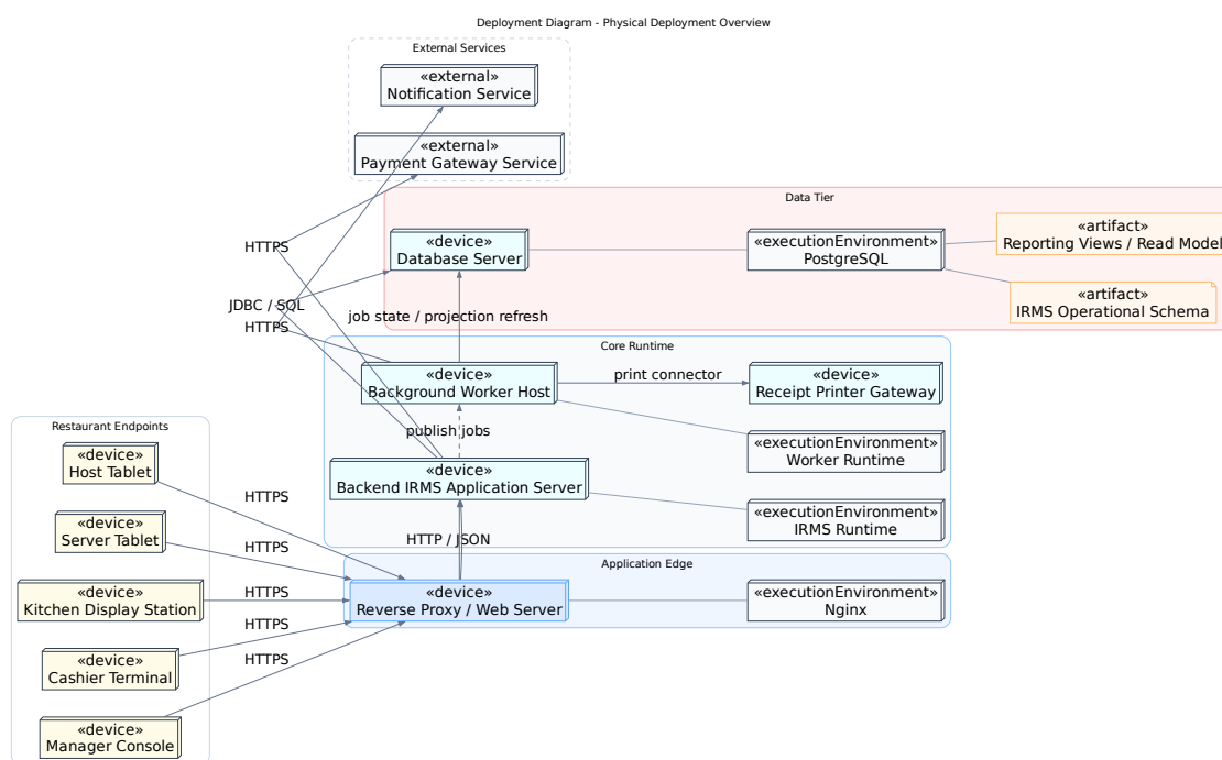
Hình 23: Sơ đồ triển khai tổng quan về bố trí vật lý của IRMS
