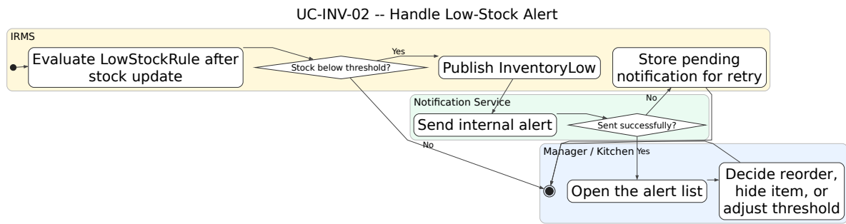
Hình 55: Sơ đồ hoạt động cho UC-INV-02 – Nhận cảnh báo sắp hết hàng
