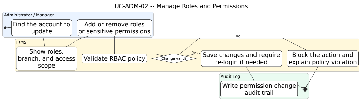
Hình 59: Sơ đồ hoạt động cho UC-ADM-02 – Quản lý vai trò và phân quyền
