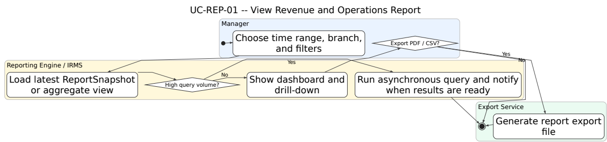
Hình 57: Sơ đồ hoạt động cho UC-REP-01 – Xem báo cáo doanh thu và vận hành
