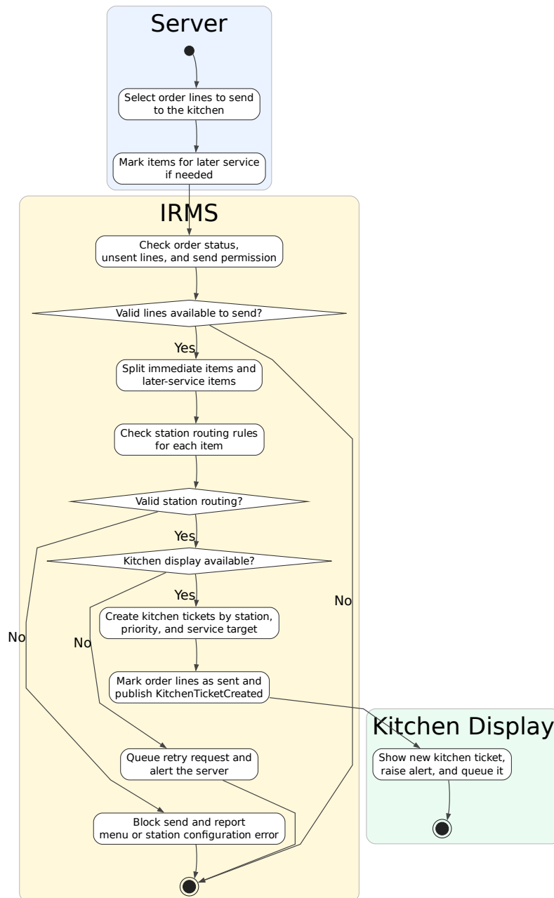
Hình 44: Sơ đồ hoạt động cho UC-ORD-03 – Gửi đơn gọi món sang bếp
