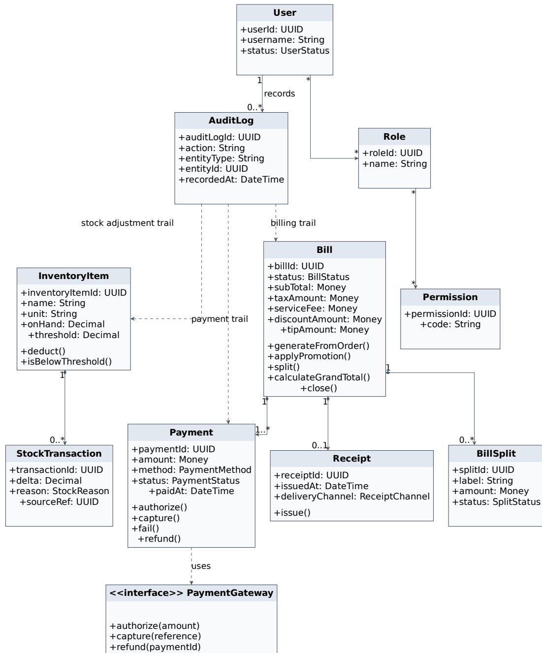
Hình 30: Sơ đồ lớp UML của cụm thanh toán, tồn kho và quản trị
