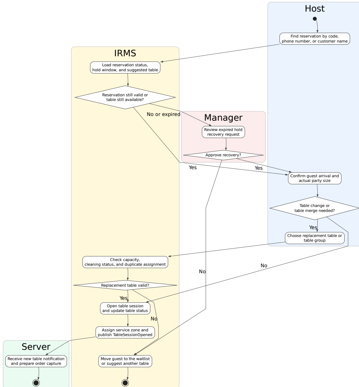
Hình 38: Sơ đồ hoạt động cho UC-RES-02 – Nhận khách và sắp bàn
