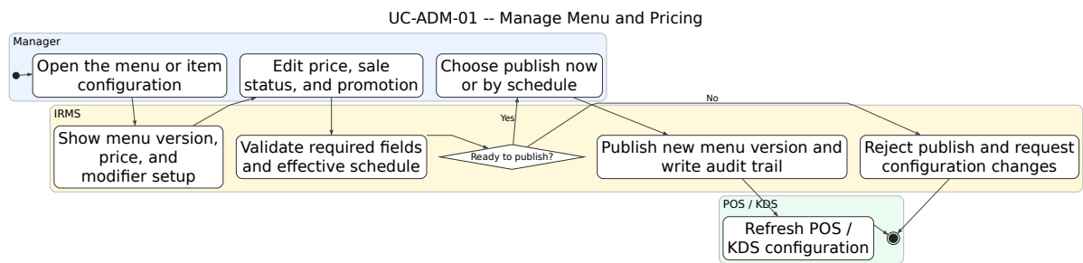
Hình 58: Sơ đồ hoạt động cho UC-ADM-01 – Quản lý thực đơn và giá bán
