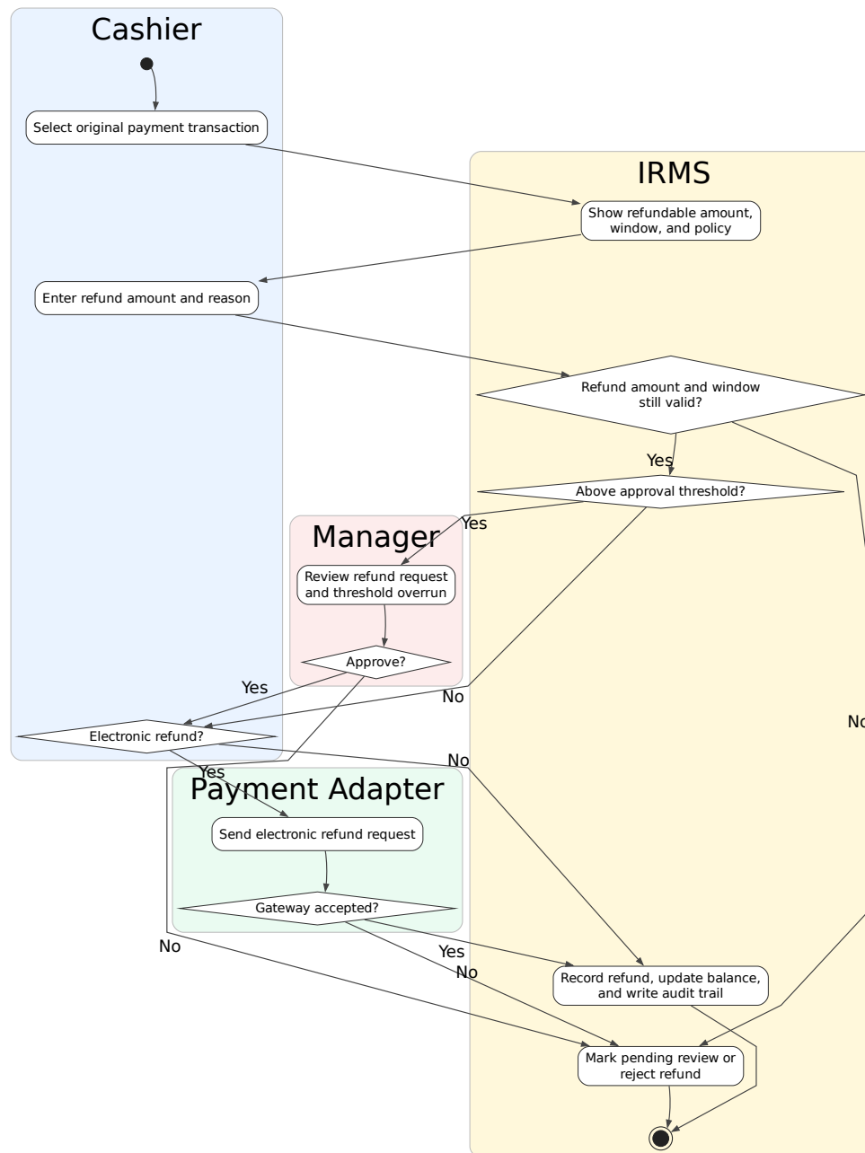
Hình 53: Sơ đồ hoạt động cho UC-PAY-03 – Hoàn tiền
