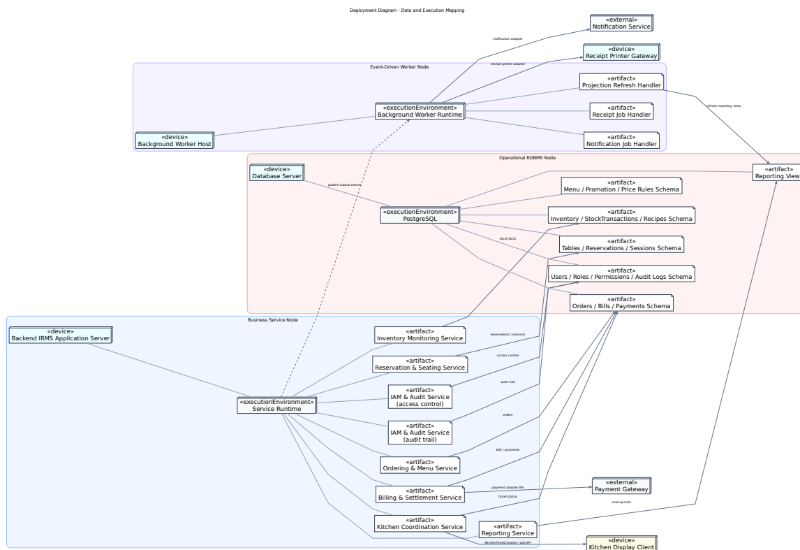
Hình 25: Sơ đồ triển khai về ánh xạ dữ liệu và thực thi
