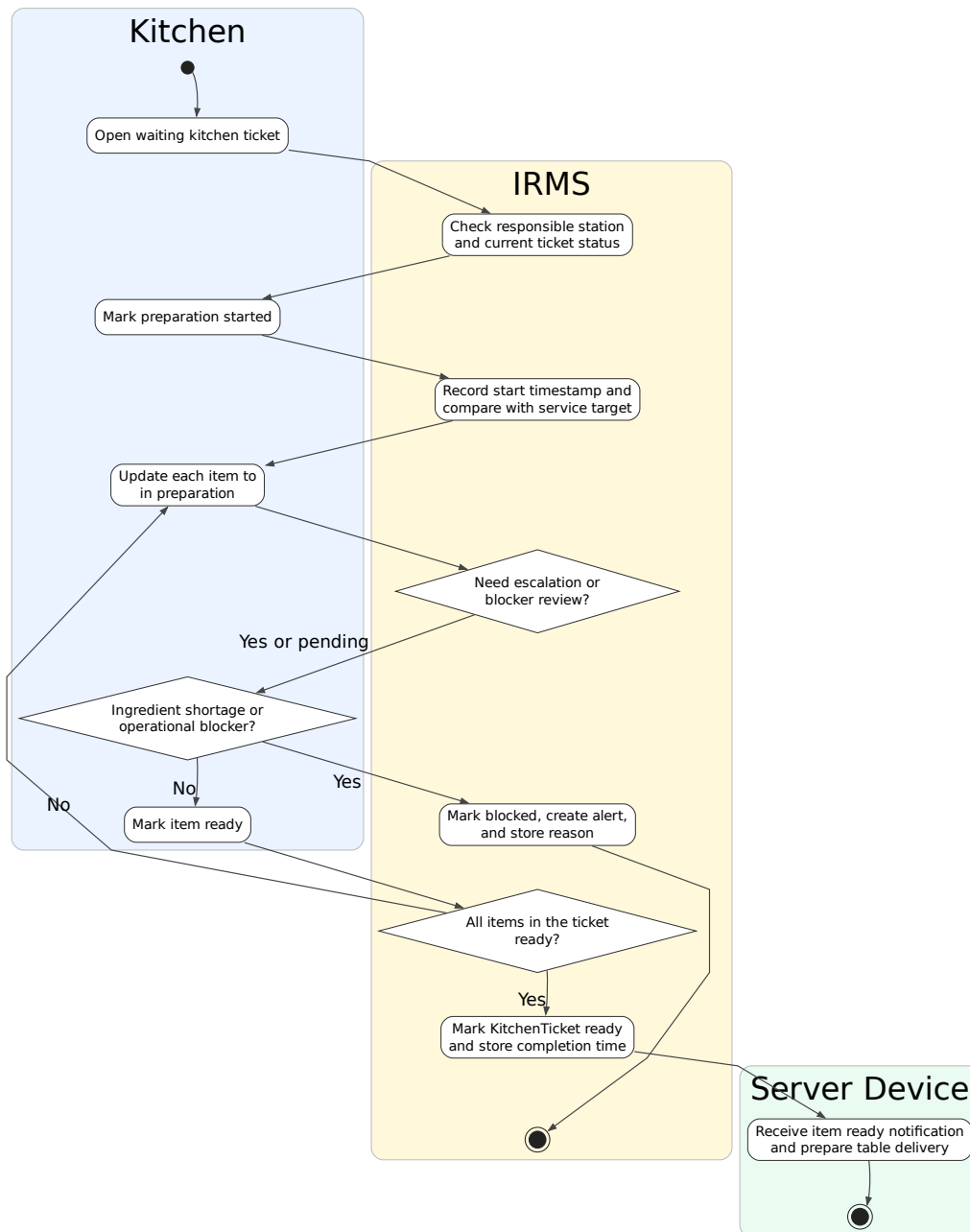
Hình 45: Sơ đồ hoạt động cho UC-KIT-01 – Cập nhật tiến độ chế biến
