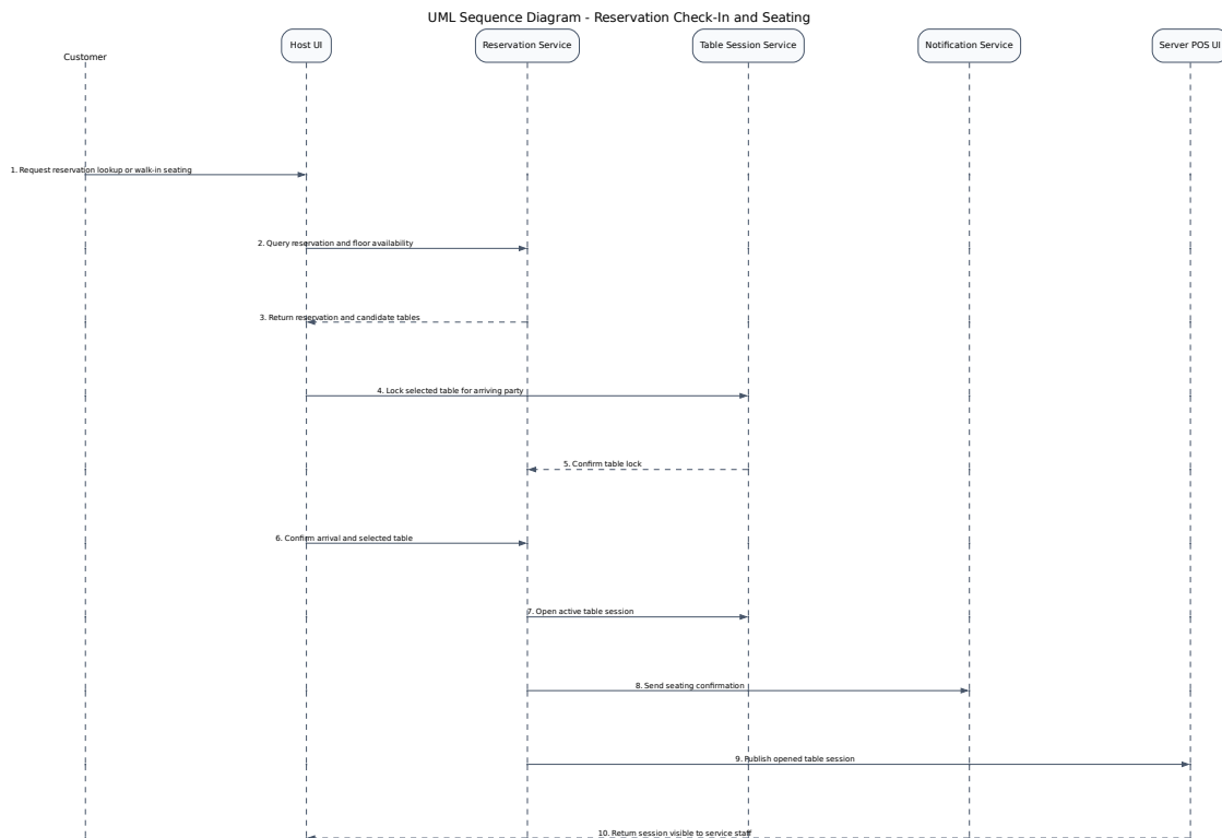
Hình 4: Sơ đồ trình tự cho kịch bản từ đặt bàn đến tiếp nhận và xếp bàn
