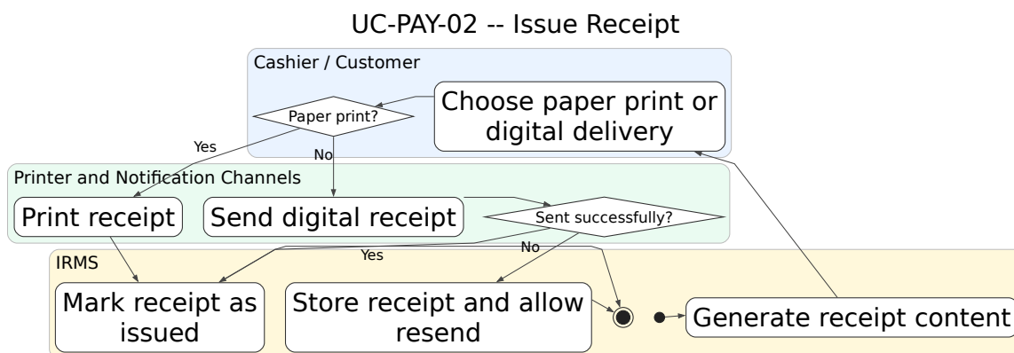
Hình 52: Sơ đồ hoạt động cho UC-PAY-02 – Phát hành biên lai
