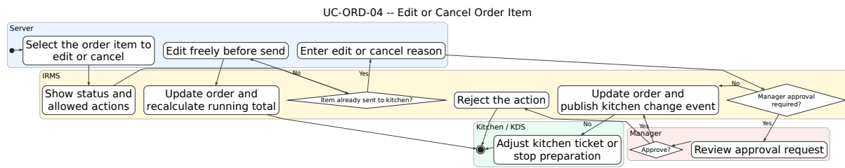
Hình 48: Sơ đồ hoạt động cho UC-ORD-04 – Sửa hoặc hủy dòng món
