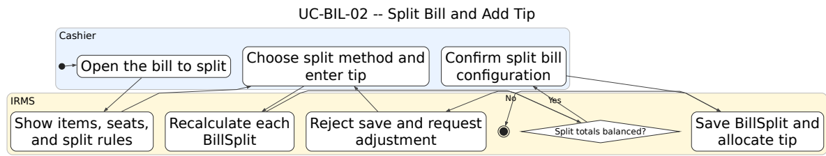
Hình 50: Sơ đồ hoạt động cho UC-BIL-02 – Tách hóa đơn và thêm tiền boa
