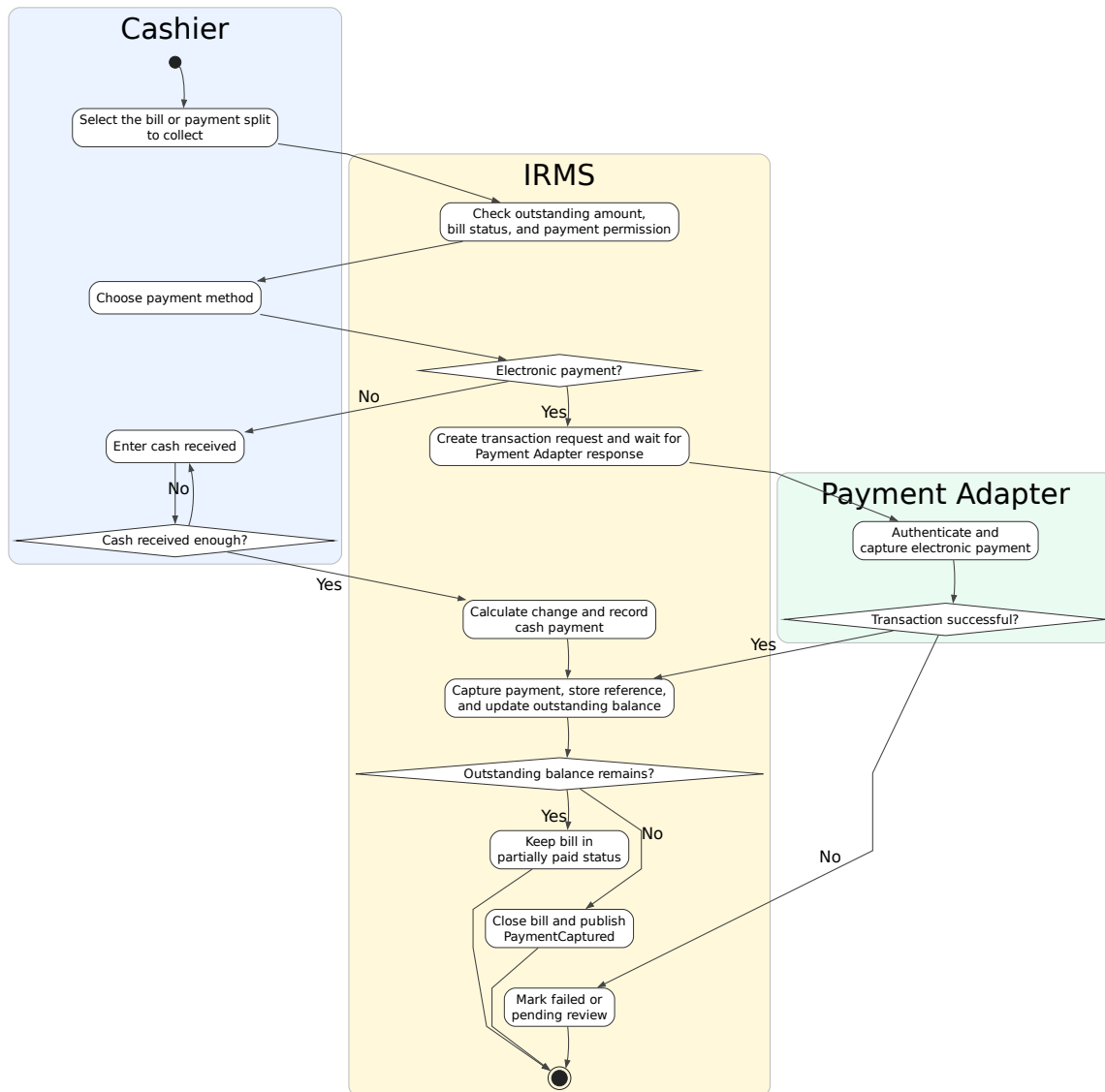
Hình 51: Sơ đồ hoạt động cho UC-PAY-01 – Xử lý thanh toán
