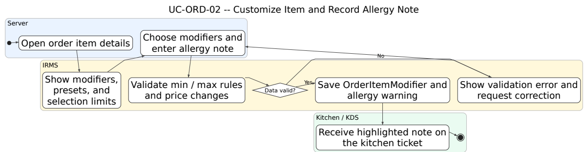
Hình 43: Sơ đồ hoạt động cho UC-ORD-02 – Tùy biến món và ghi chú dị ứng
