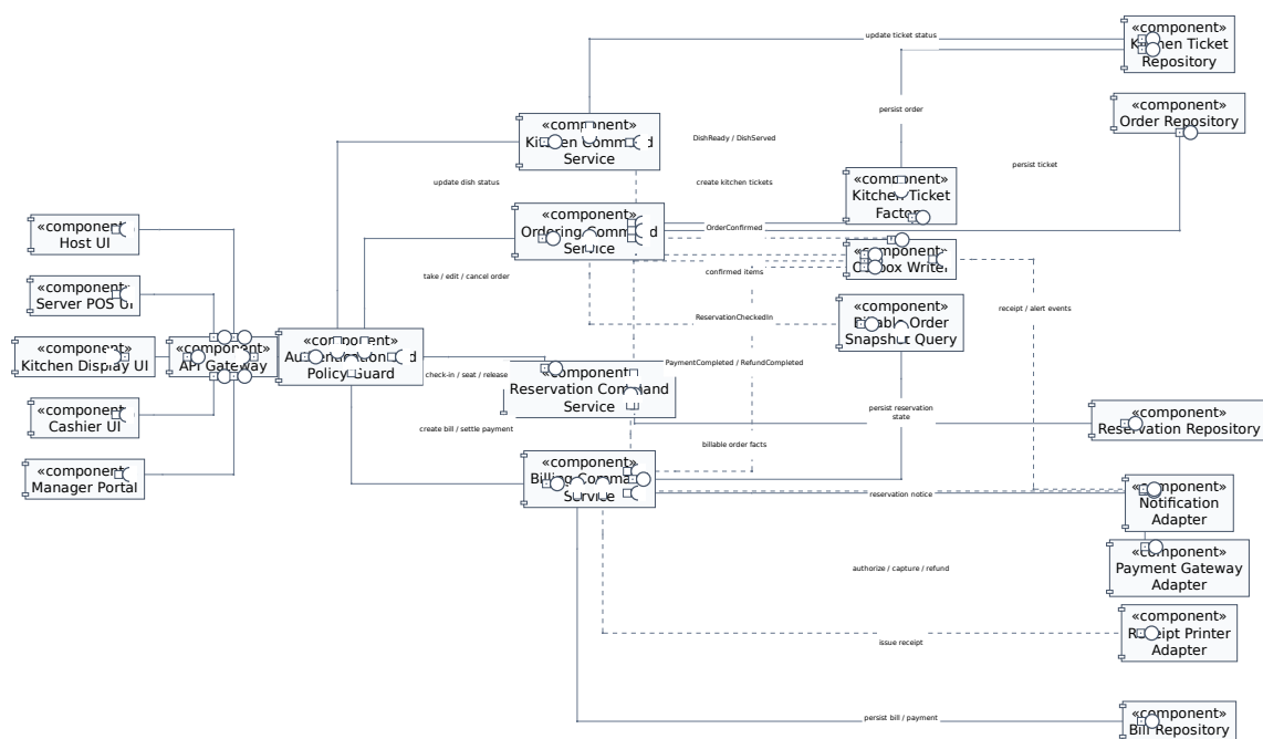
Hình 21: Sơ đồ thành phần cho tuyến lệnh vận hành của IRMS
