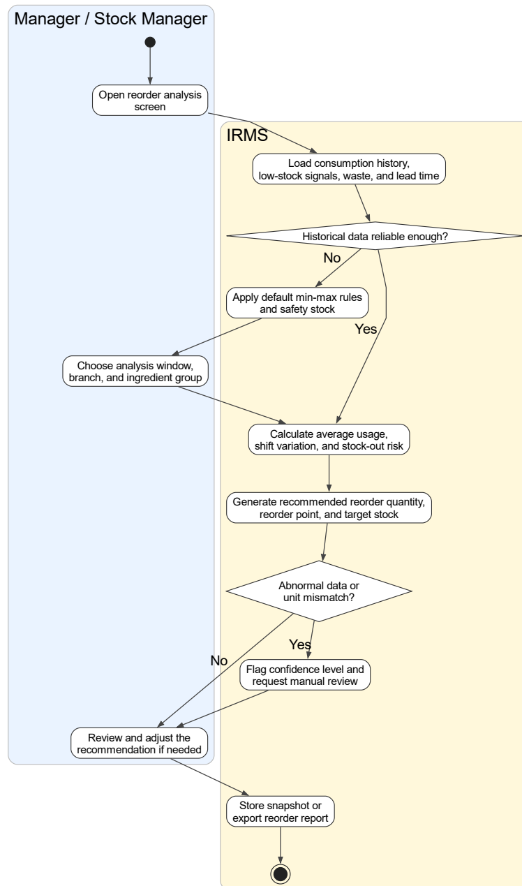
Hình 56: Sơ đồ hoạt động cho UC-INV-03 – Phân tích tiêu hao và đề xuất nhập hàng
