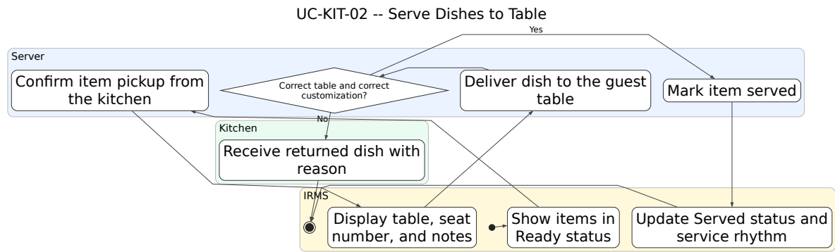
Hình 46: Sơ đồ hoạt động cho UC-KIT-02 – Ra món cho bàn
