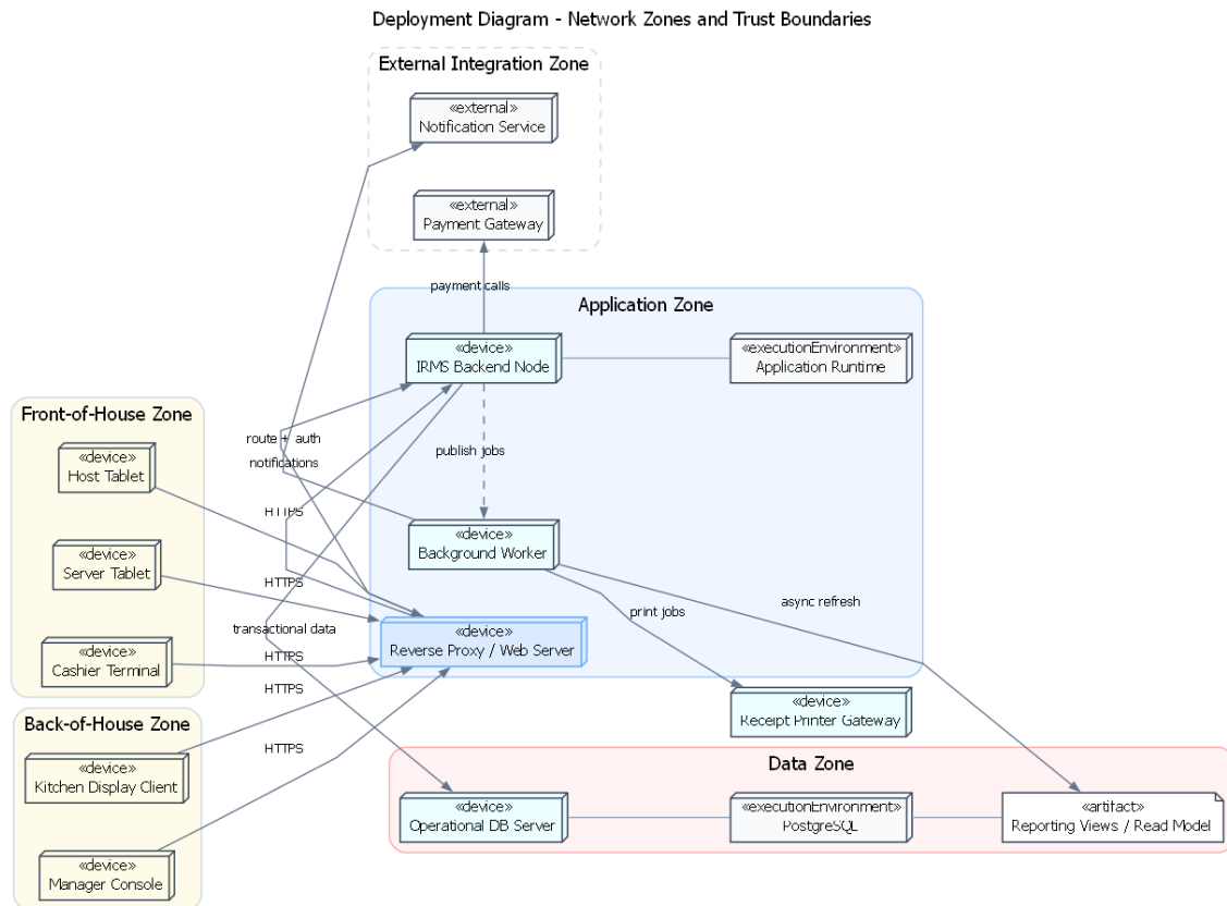
Hình 24: Sơ đồ triển khai theo vùng mạng và ranh giới tin cậy
