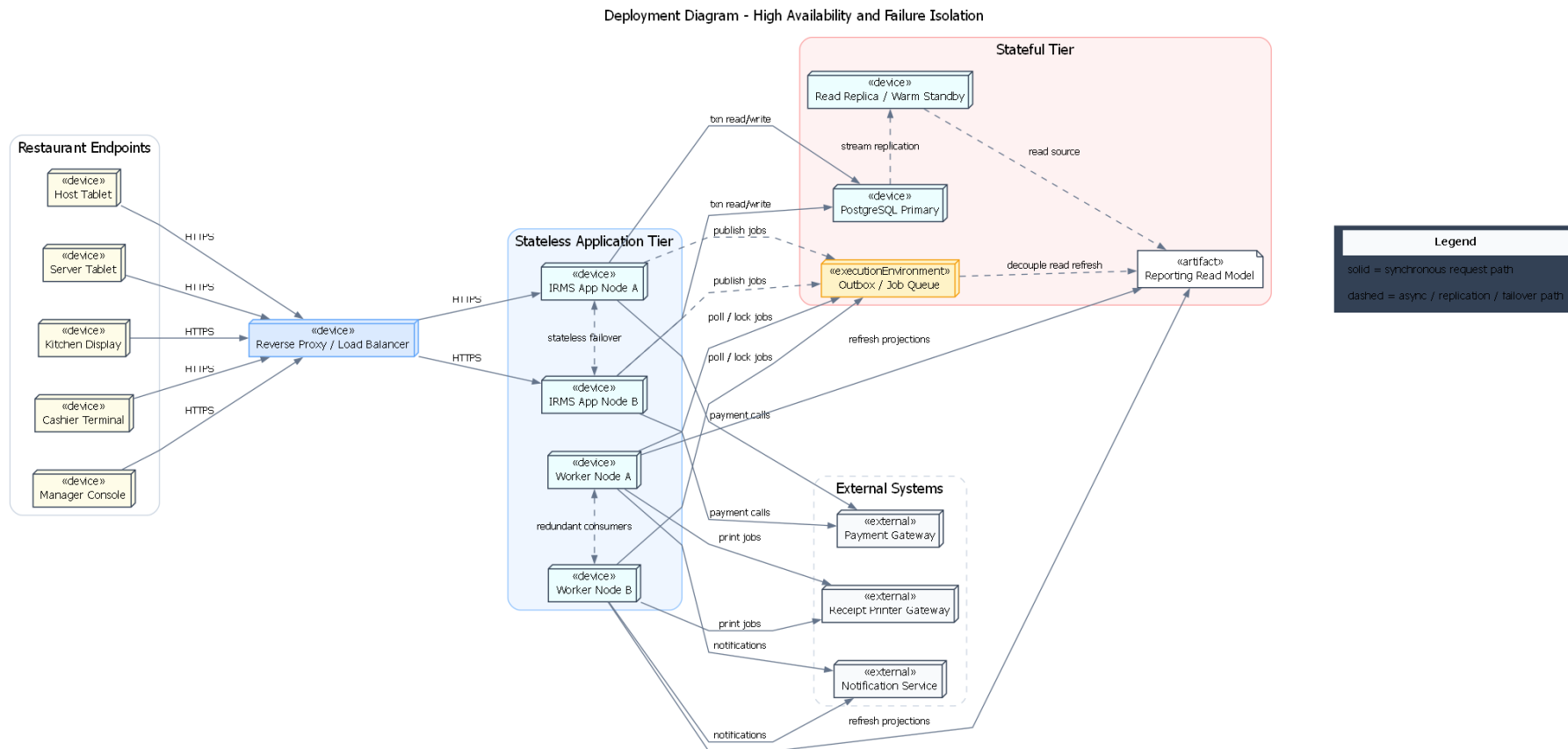
Hình 26: Sơ đồ triển khai cho tính sẵn sàng cao và cô lập lỗi
