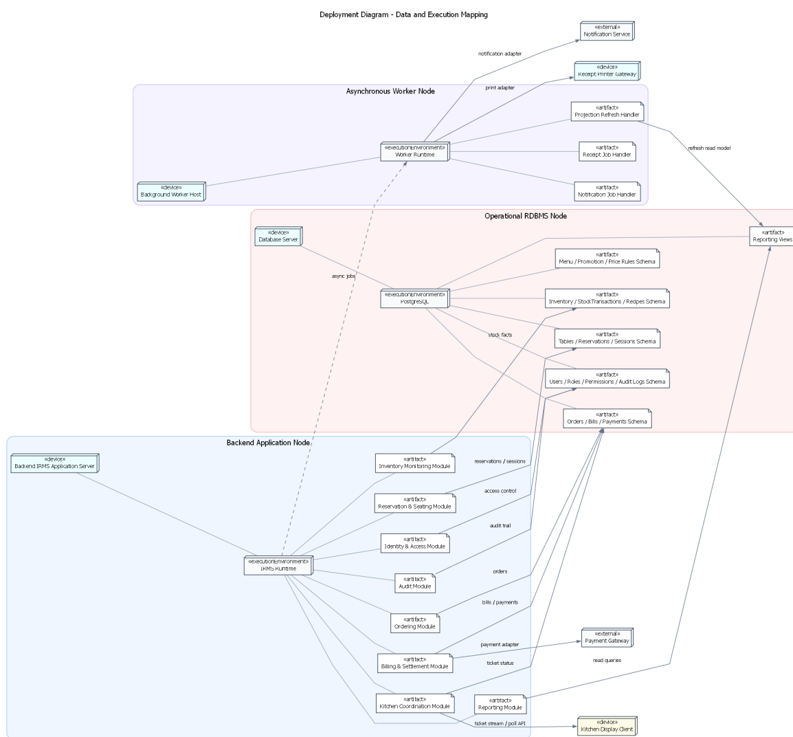
Hình 25: Sơ đồ triển khai về ánh xạ dữ liệu và thực thi
