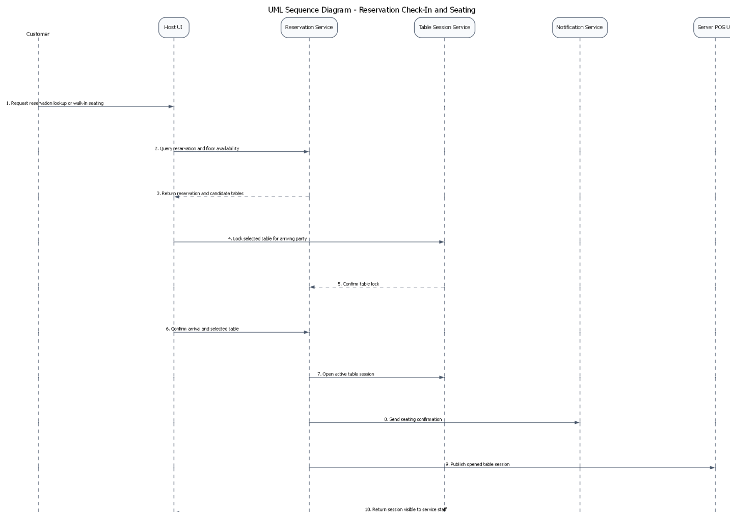
Hình 4: Sơ đồ trình tự cho kịch bản từ đặt bàn đến tiếp nhận và xếp bàn
