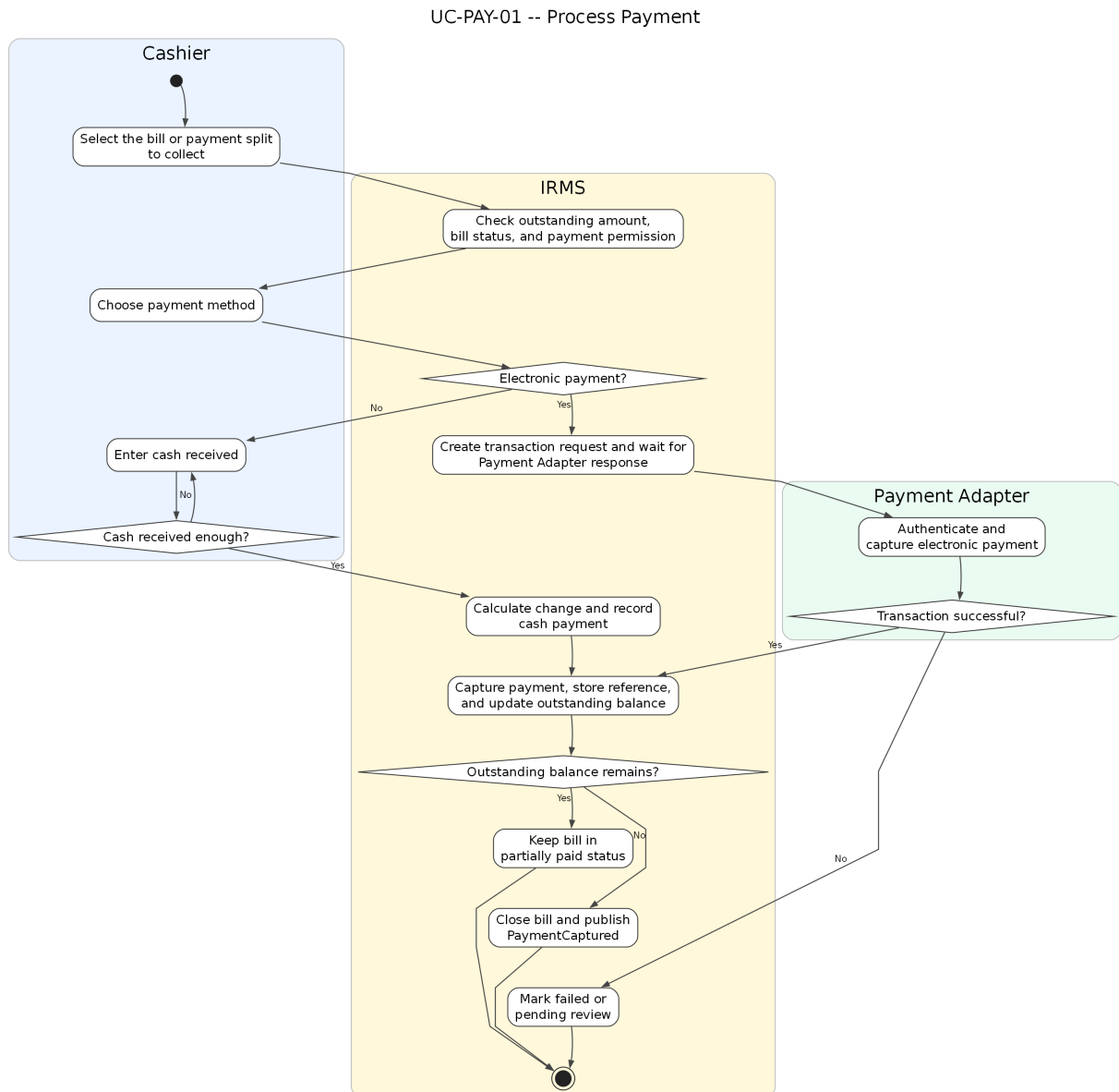
Hình 51: Sơ đồ hoạt động cho UC-PAY-01 – Xử lý thanh toán
