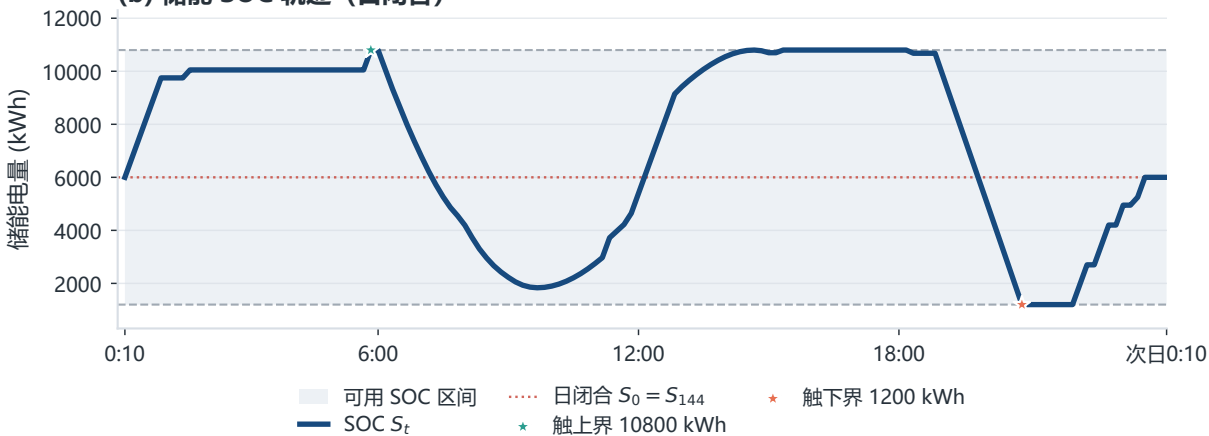
(b) 储能 SOC 轨迹 (日闭合)
