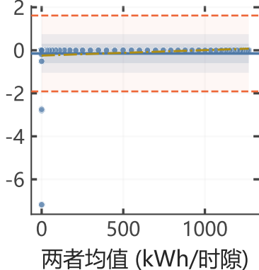
(b) 光伏
