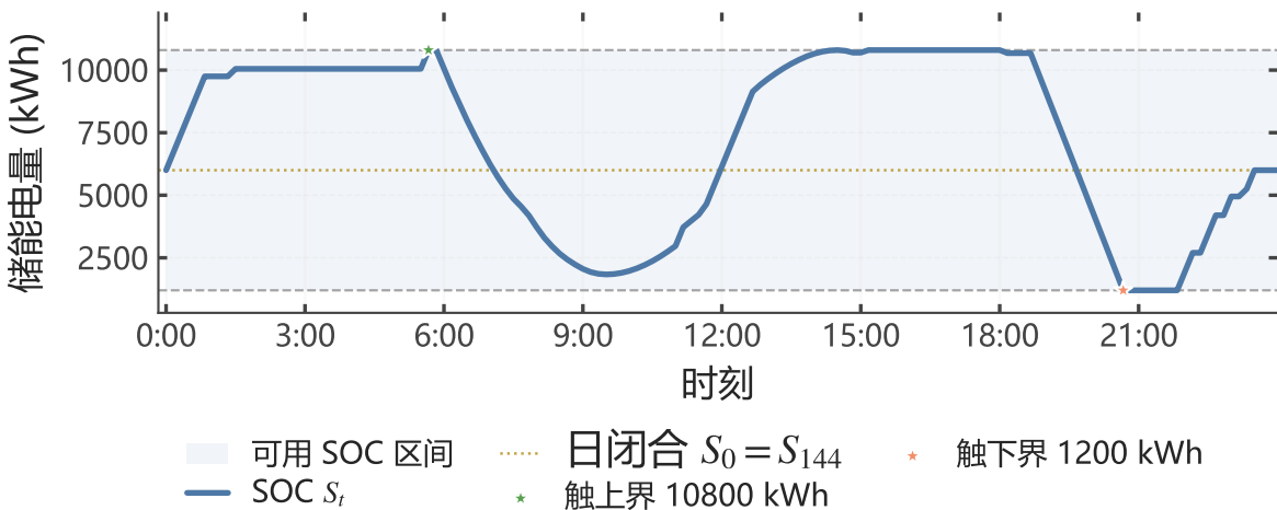
(b) 储能 SOC 轨迹 (日闭合)
