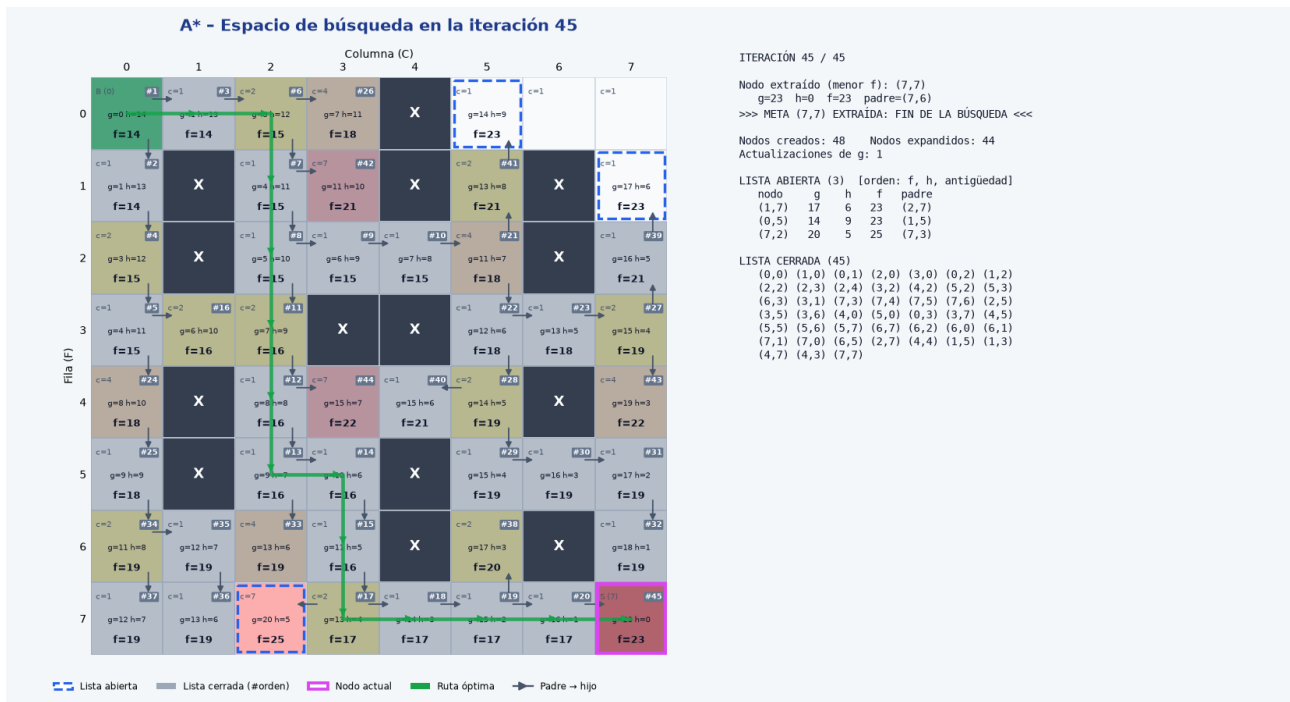
Figura 8. Última iteración (45): la meta (7,7) se extrae de la lista abierta y se dibuja la ruta óptima.
