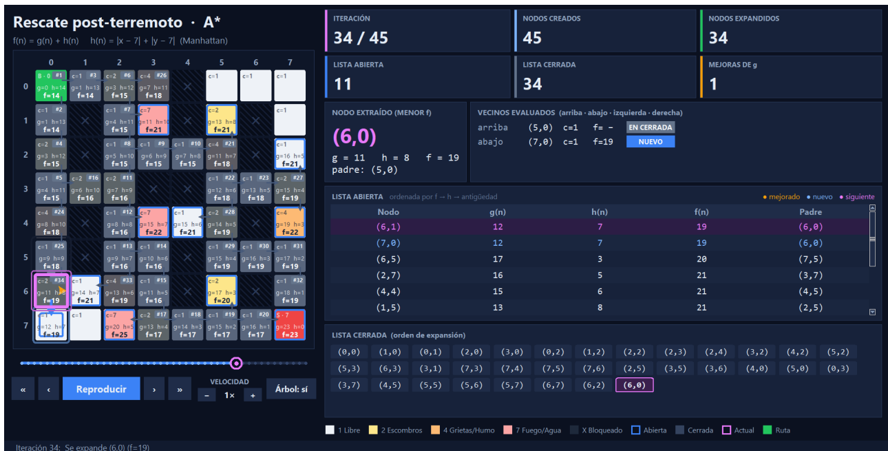
Figura 7. Interfaz animada durante la iteración 34: haces hacia los vecinos (azul = nuevo, ámbar = mejora de g) y listas abierta y cerrada.
