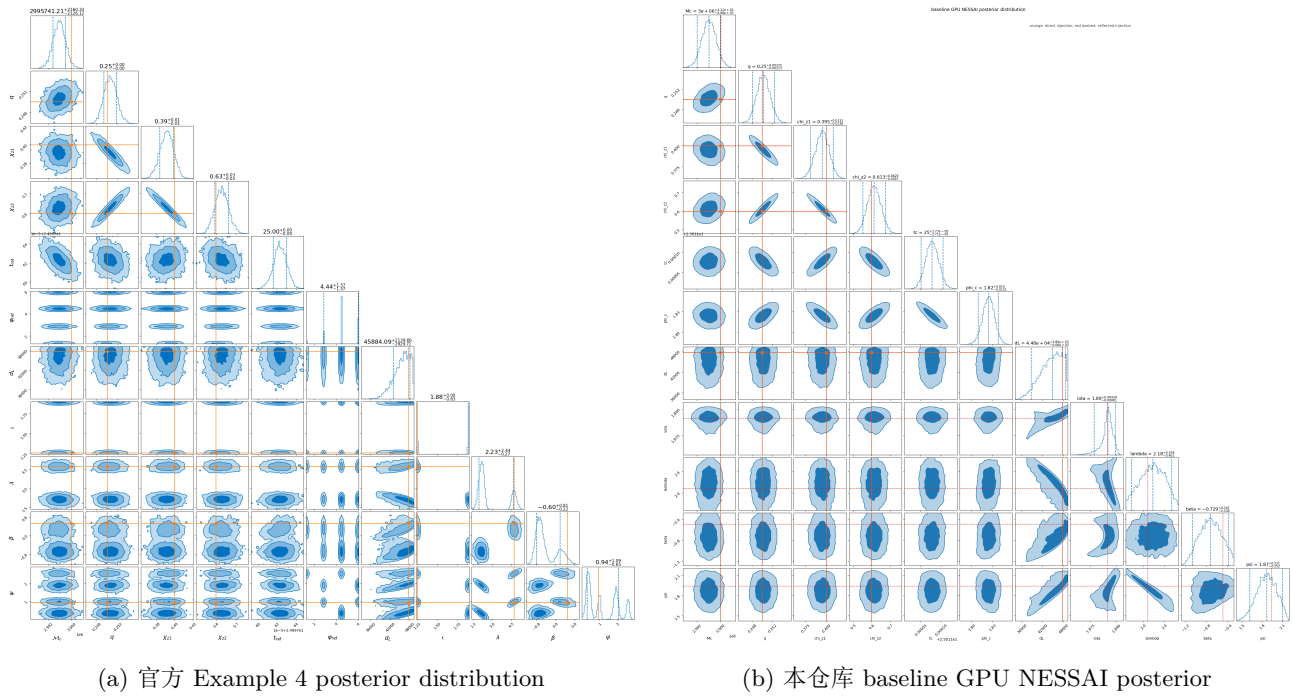
图 9: posterior distribution 对比。官方图展示 Example 4 CPU 路线下的 posterior/corner 输出，包含更明显的多模态结构；本仓库图为 GPU 杂频似然 + local-fisher NESSAI 的反射支局部后验，橙线为 direct injection，红虚线为 reflected reference。二者回答的问题不同：官方图强调示例的全局 posterior 展示，本仓库图强调在任务窗口内对反射支进行快速、可诊断的全量 NESSAI 估计。
