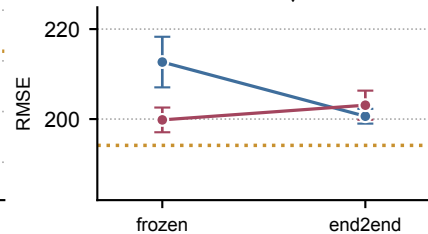
QM7 ↓
