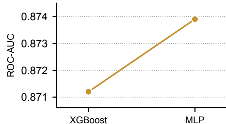
QM7 ↓
