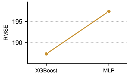
QM7 ↓
