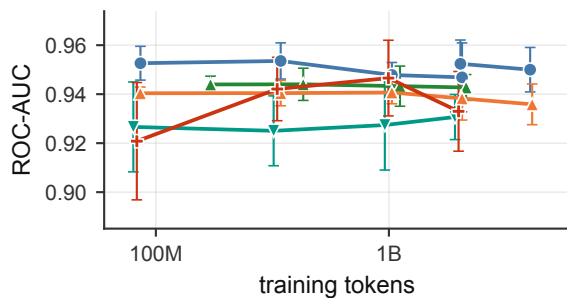
Tox21 (ROC-AUC ↑)
