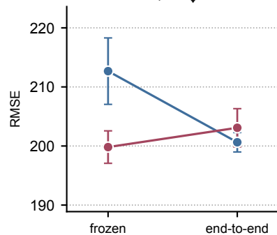
QM7 ↓
