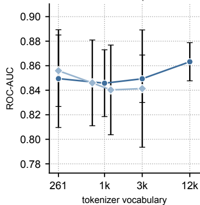
QM7 ↓
