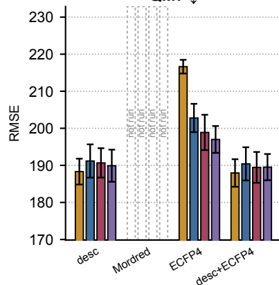
QM7 ↓
